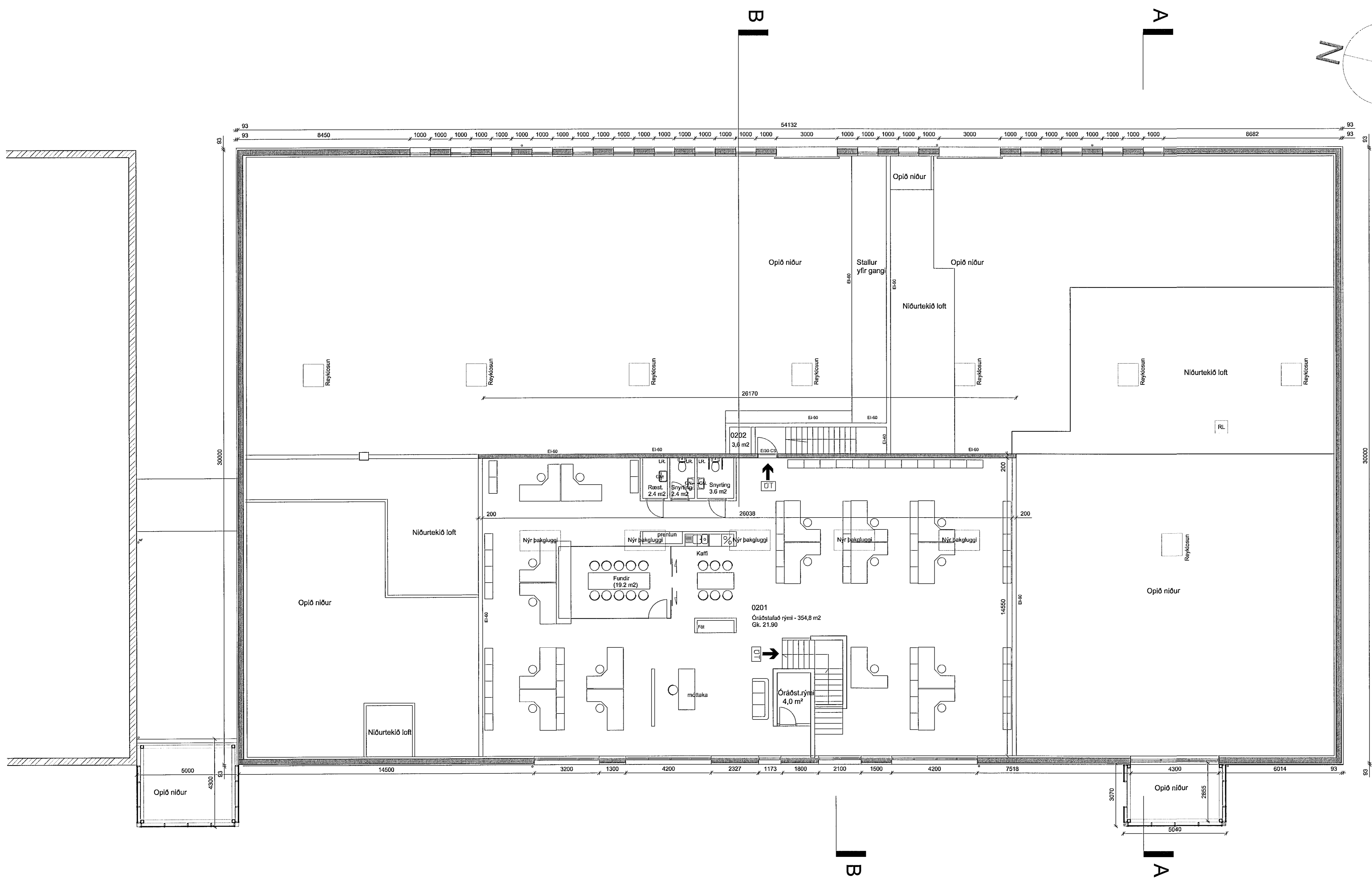
Grunnmynd 2. hæð mkv.1:200
