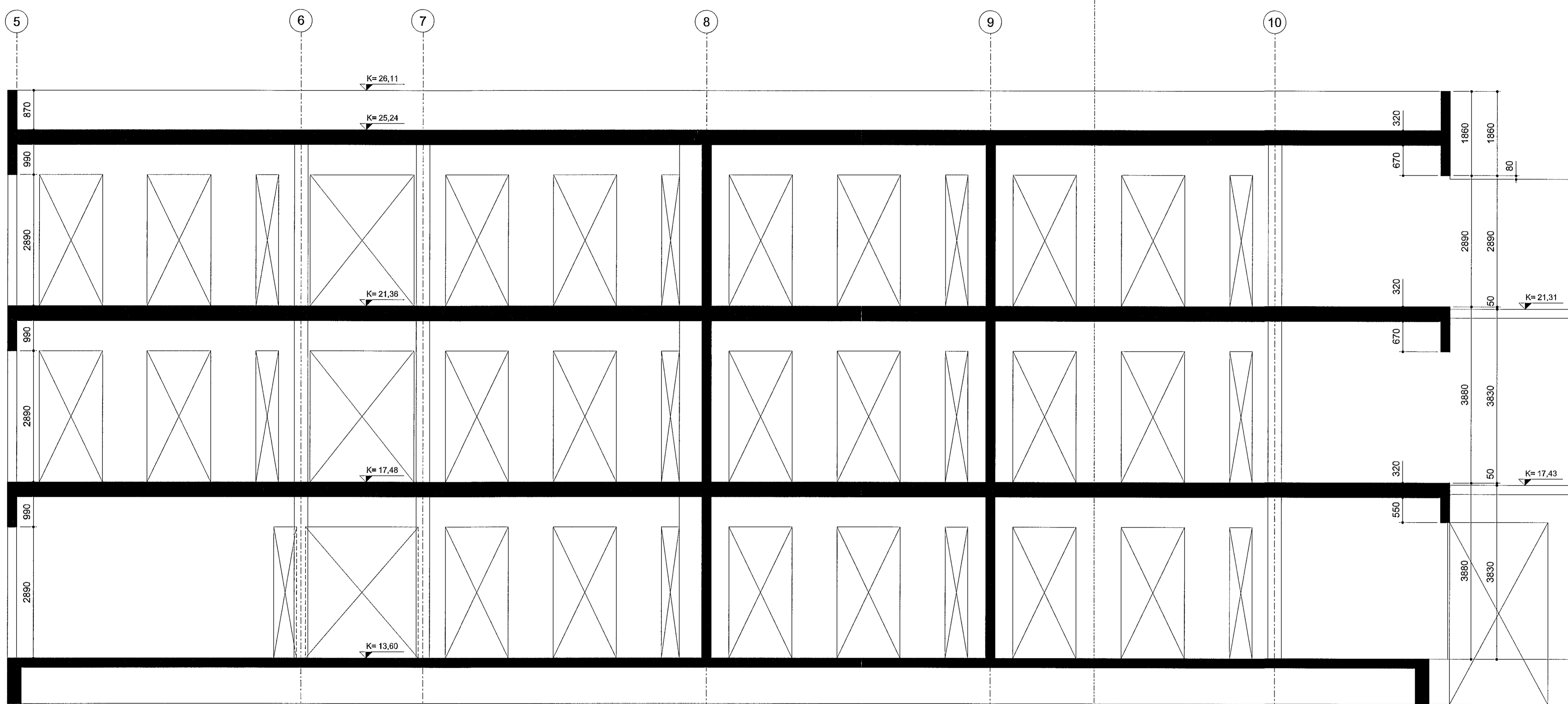
SKURÐMYND B-B NORÐUR
