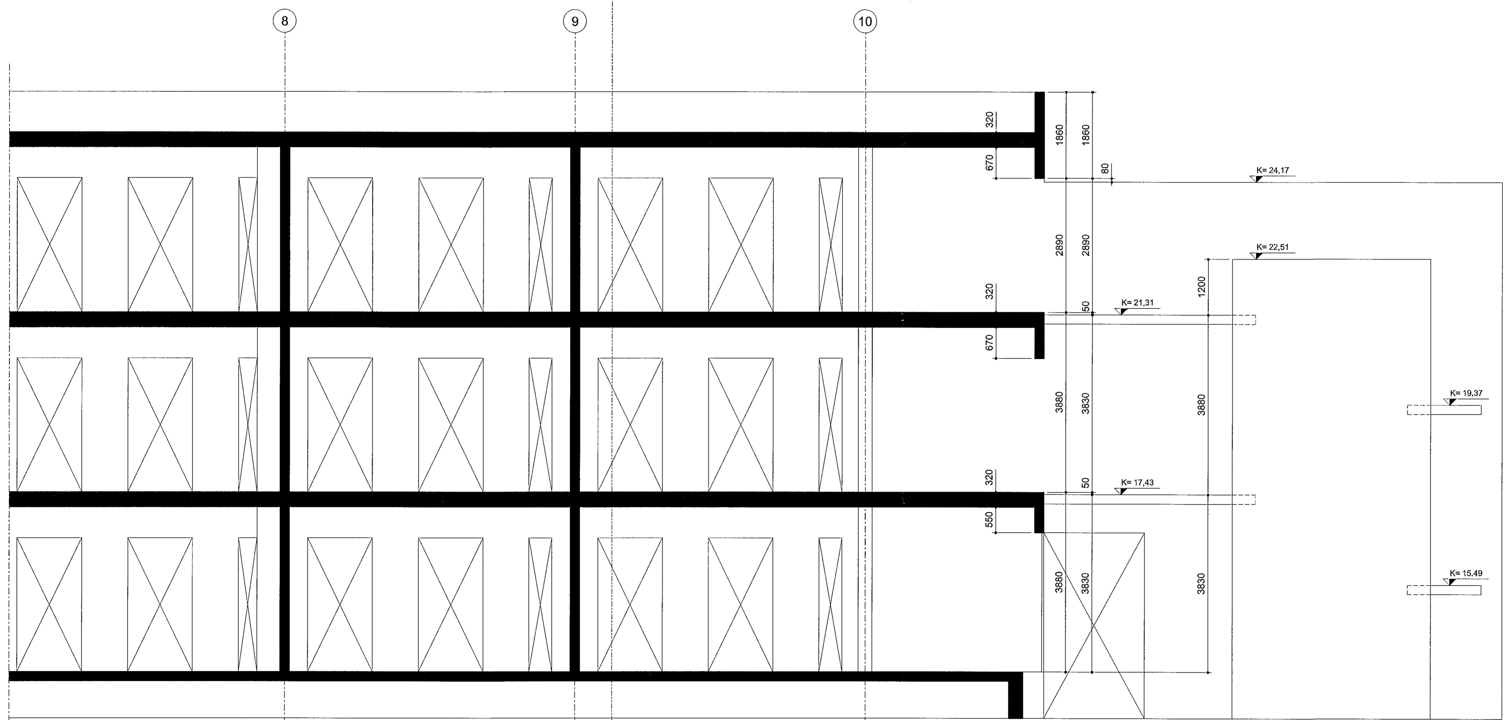
SKURÐMYND B-B SUÐUR
