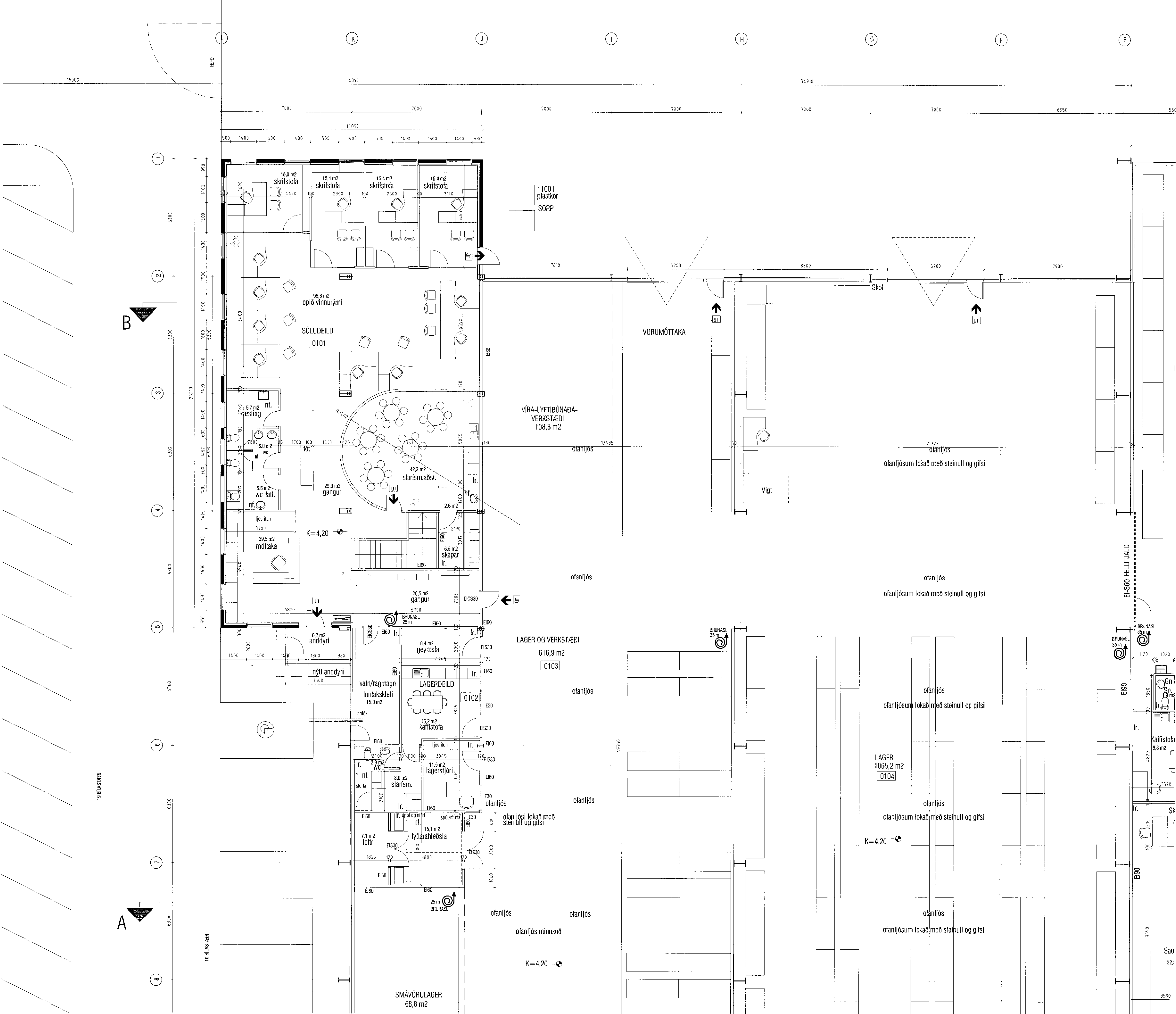
grunnmynd 1.hæð m 1:100
