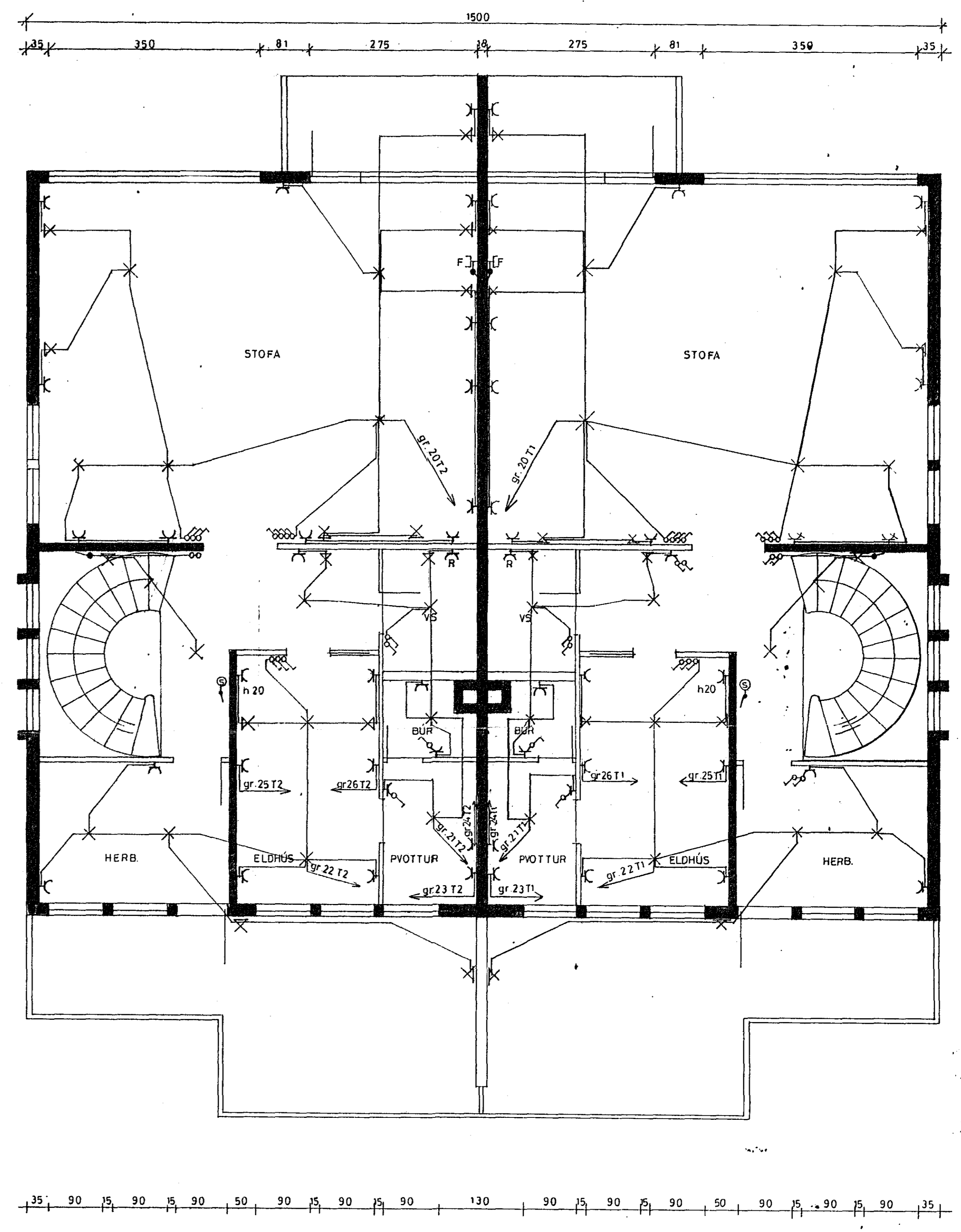
GRUNNMYND 2. HÆÐ
