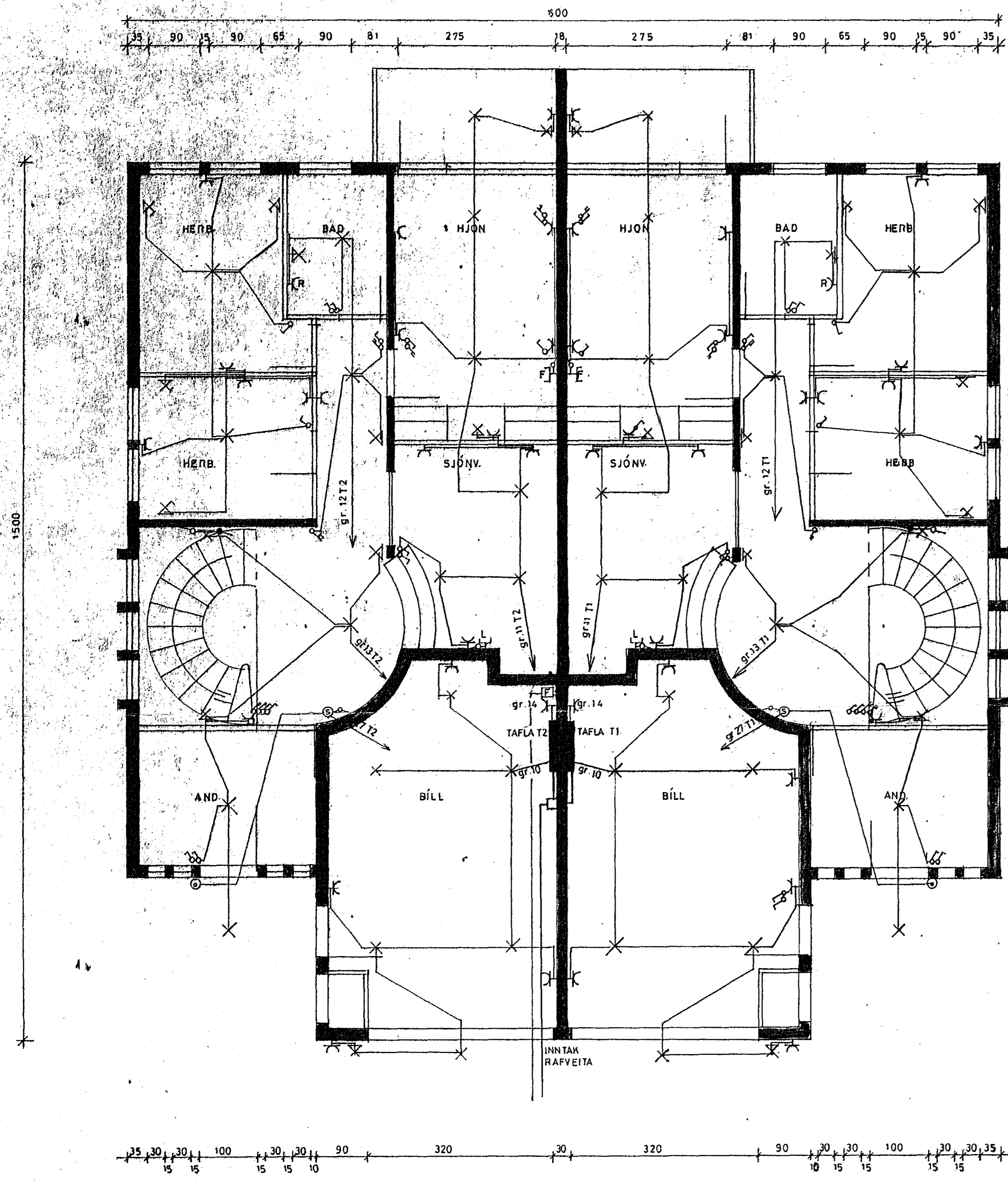
GRUNNMYND 1. HÆÐ
