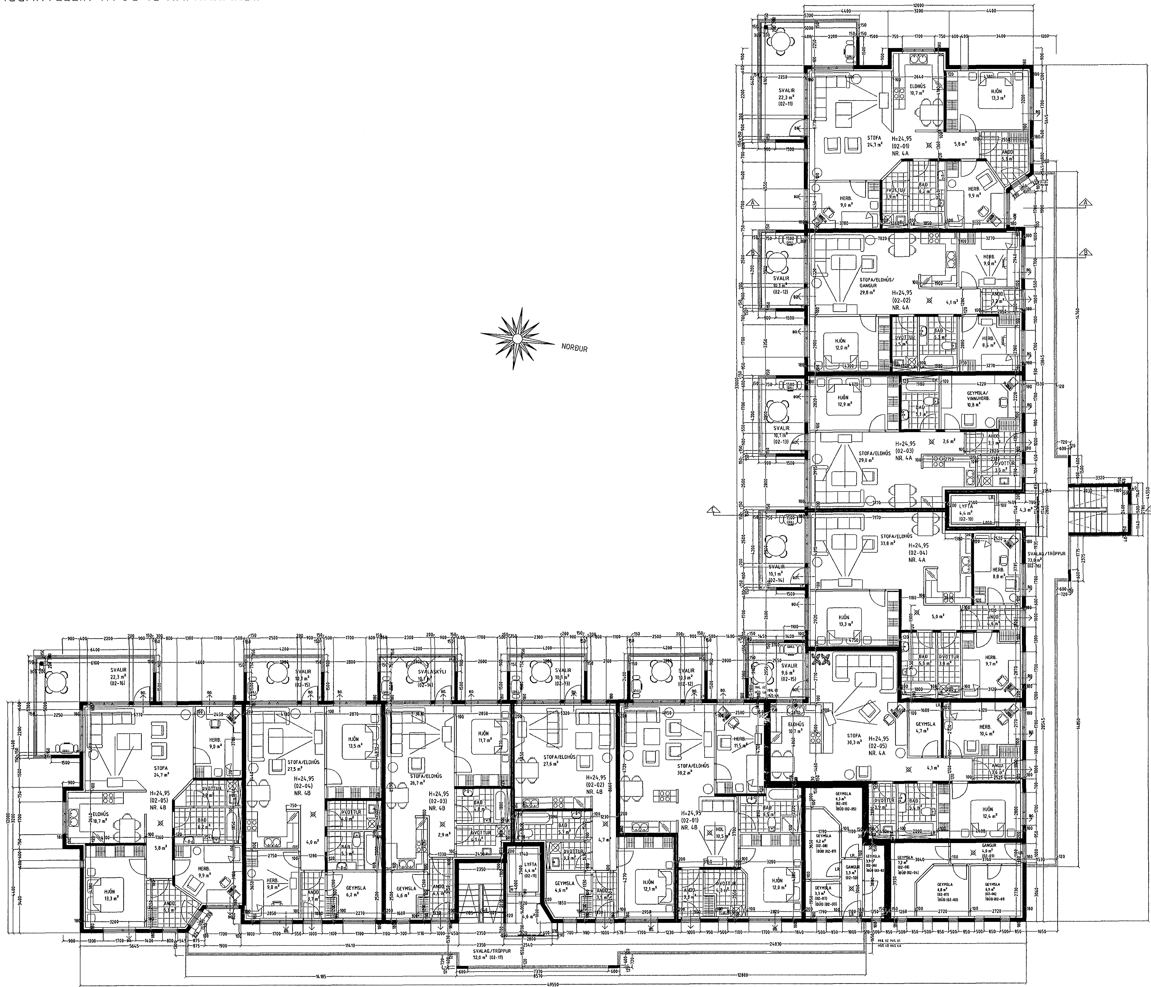
GRUNNMYND 2 HÆÐ MKV. 1:100.
