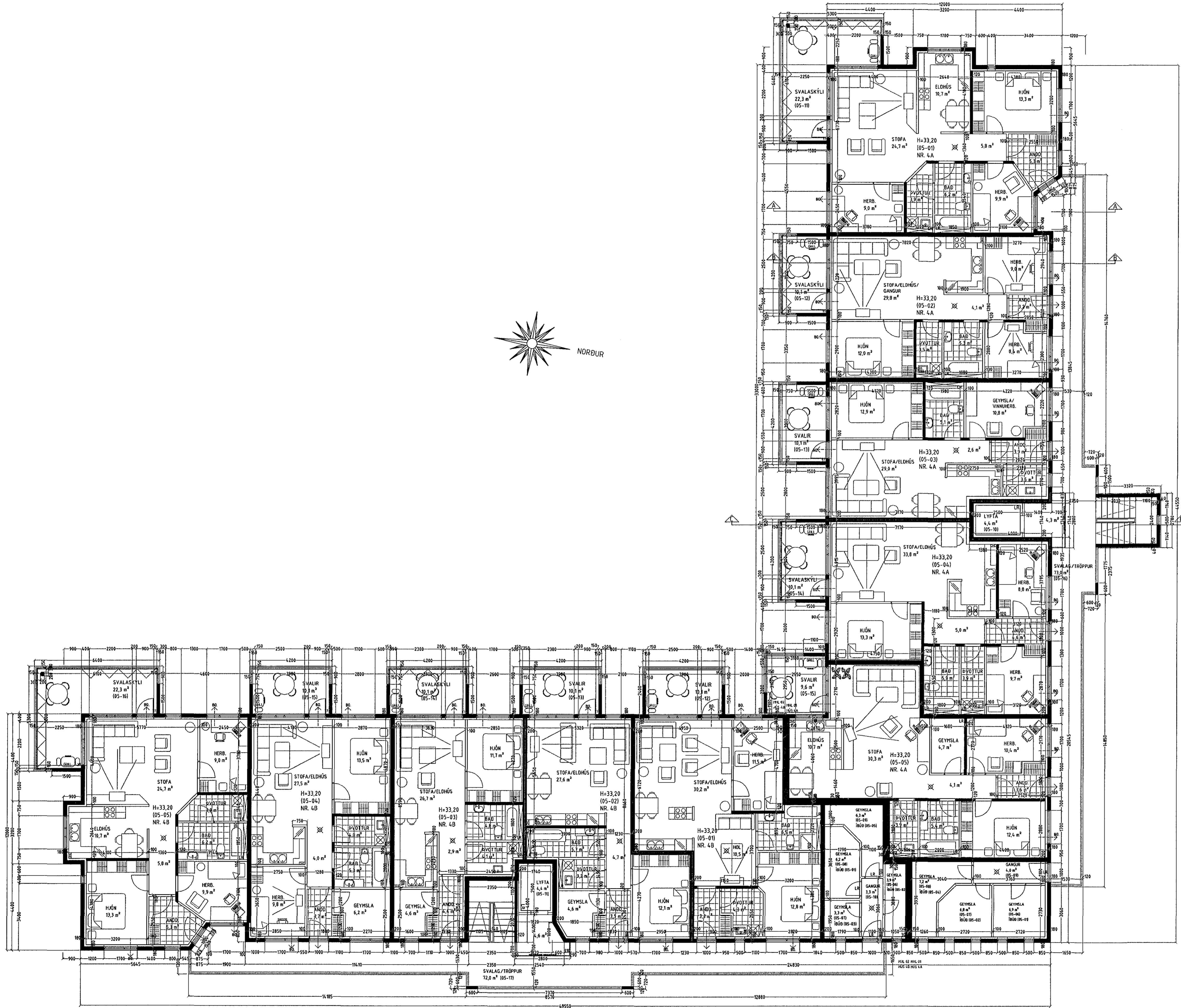
GRUNNMYND 5 HÆÐ MKV. 1:100.
