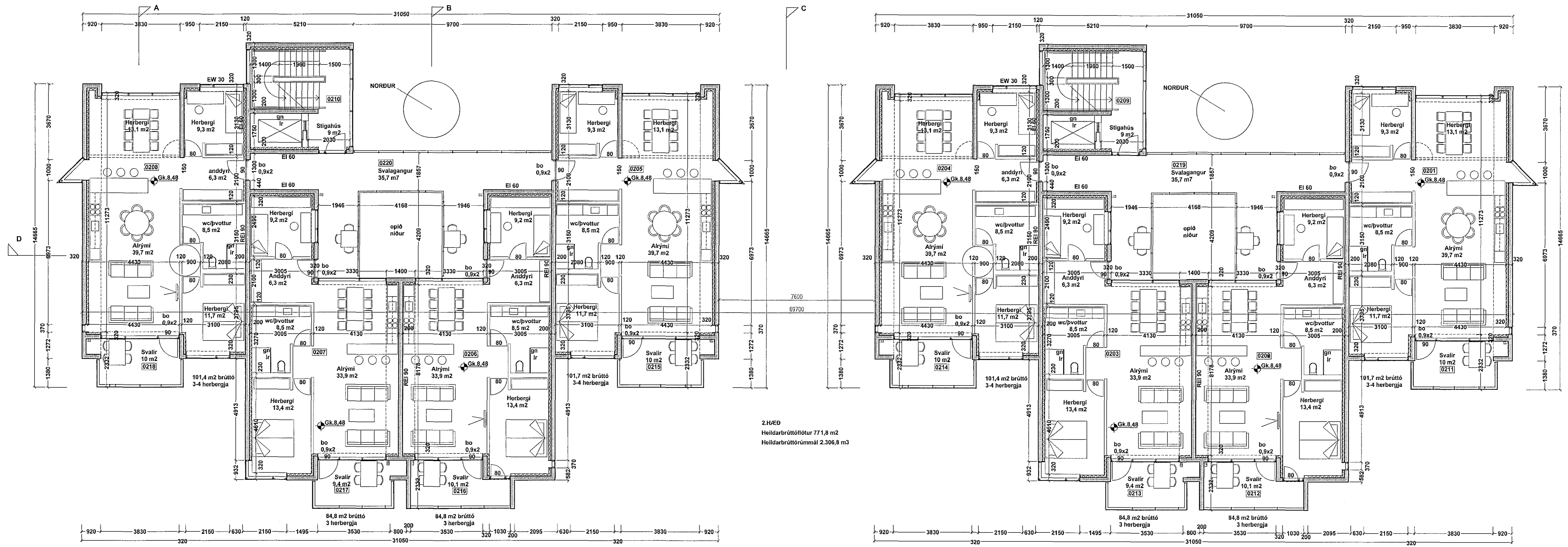
GRUNNMYND 2 HÆÐ MKV 1:100
