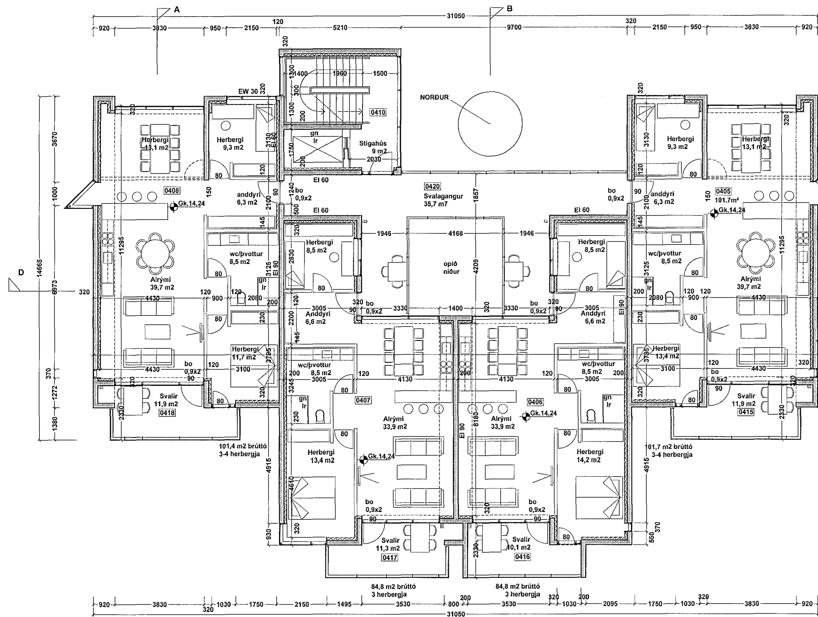
GRUNNMYND 4 HÆÐ MKV 1:100
