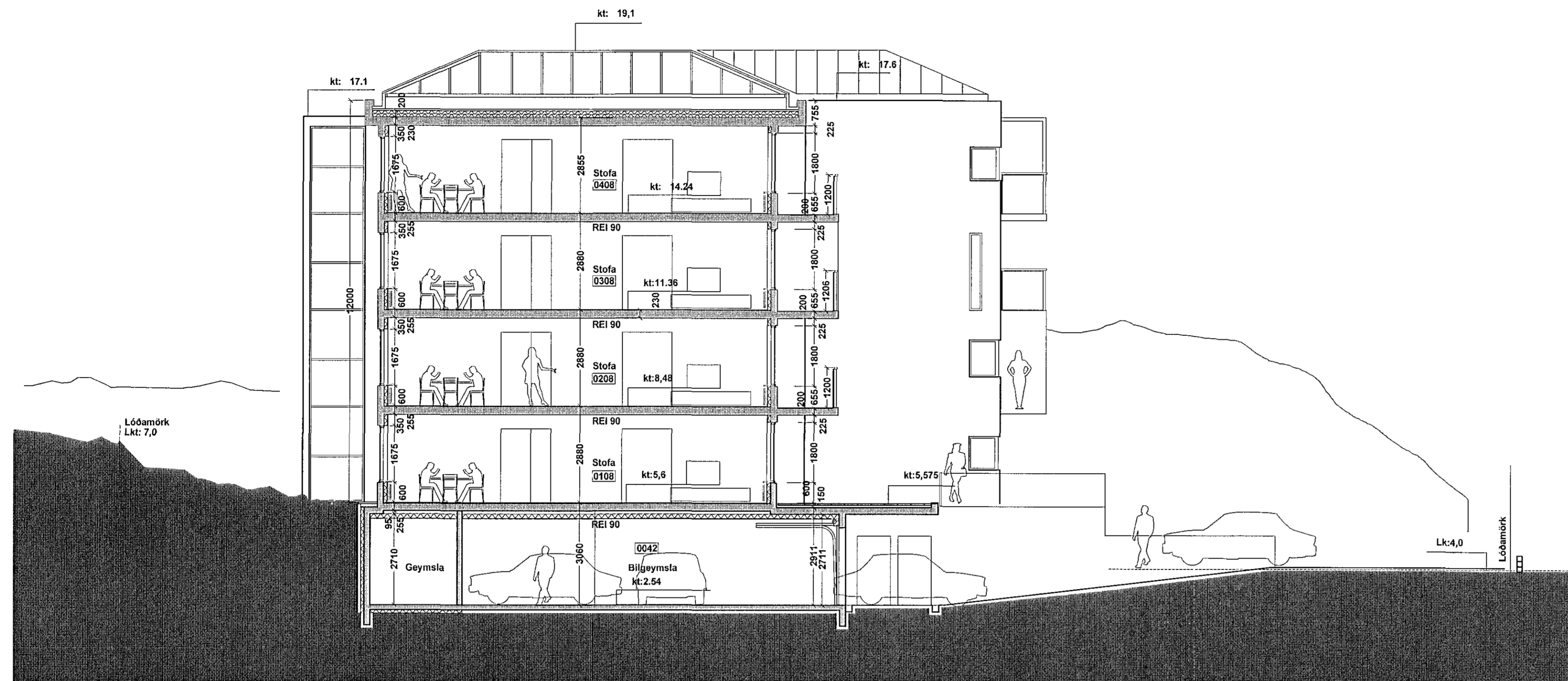
SNEIÐING A-A MKV 1:100
