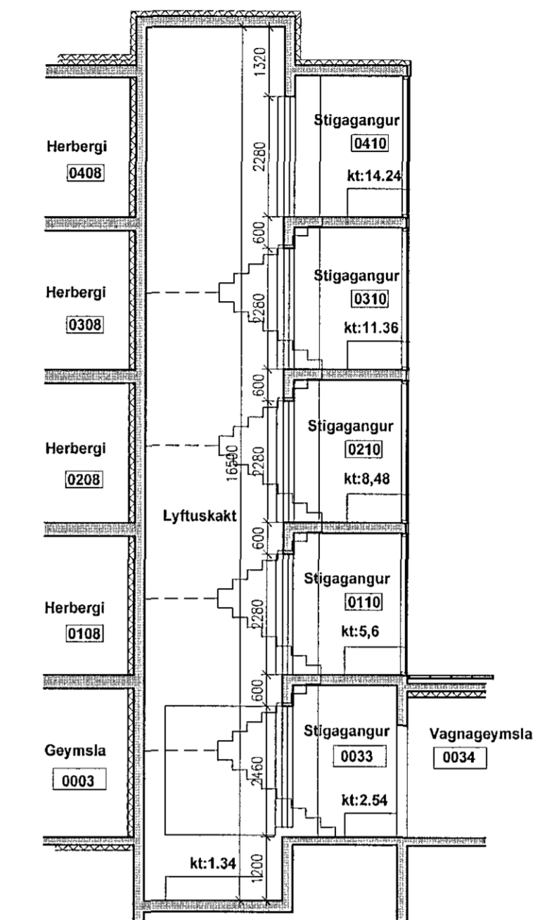
SNEIÐING Í LYFTUSKAKT MKV 1:100
