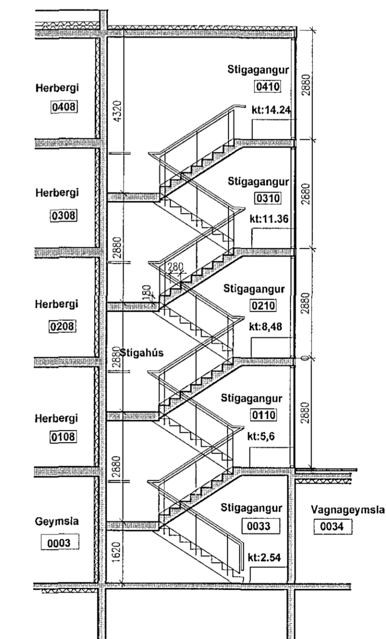
SNEIÐING Í STIGAHÚS MKV 1:100
