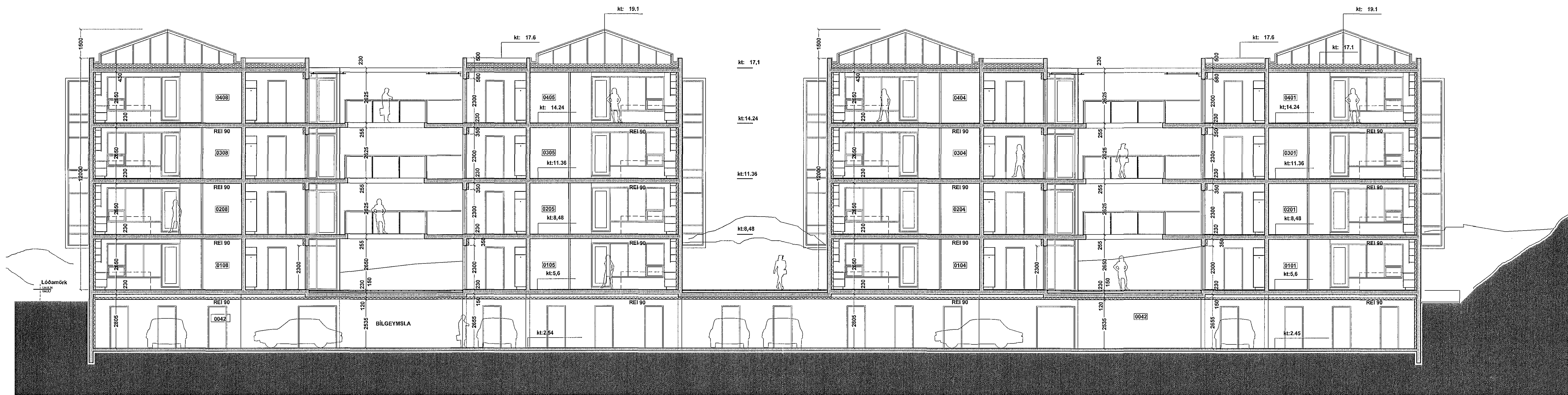
SNEIDING D-D MKV 1:100
