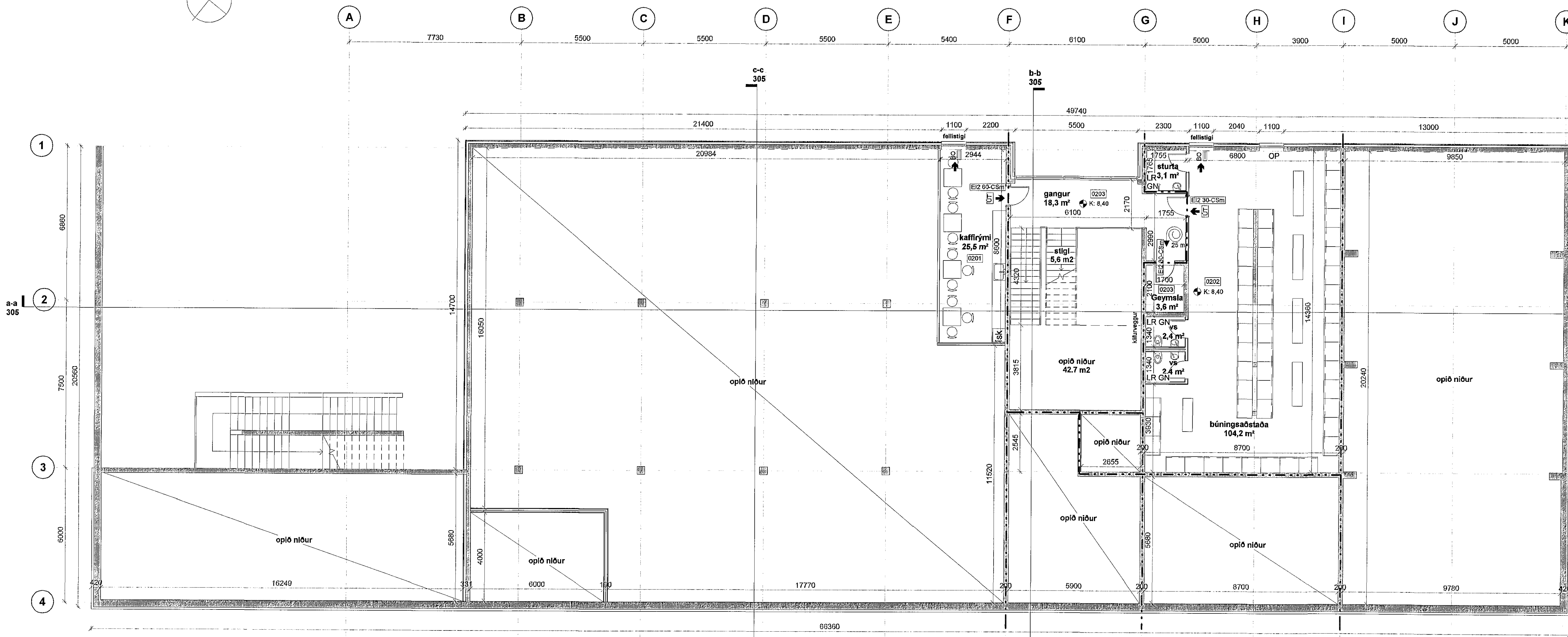
G-2. hæð 1 : 100
