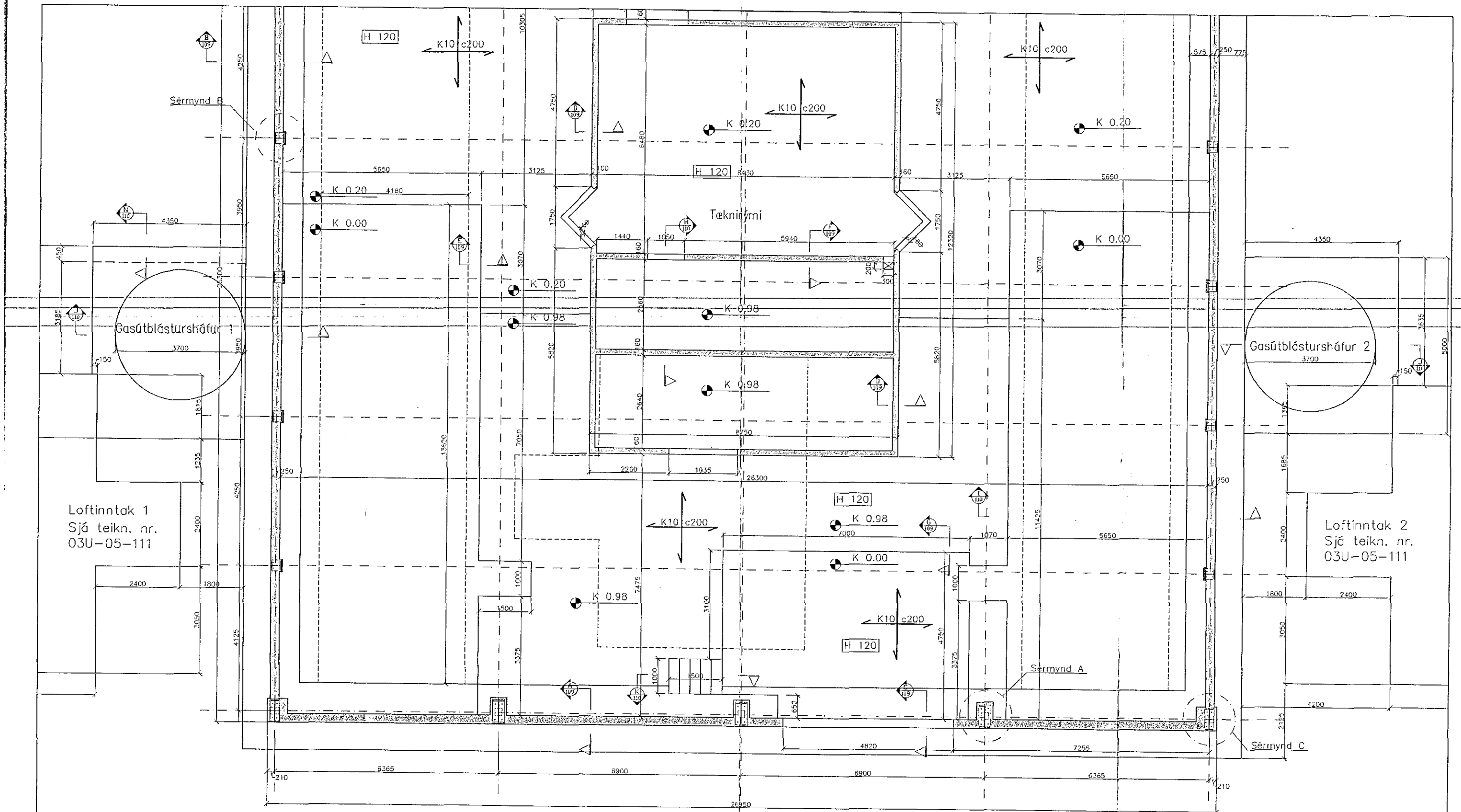
Grunnmynd 1:50
