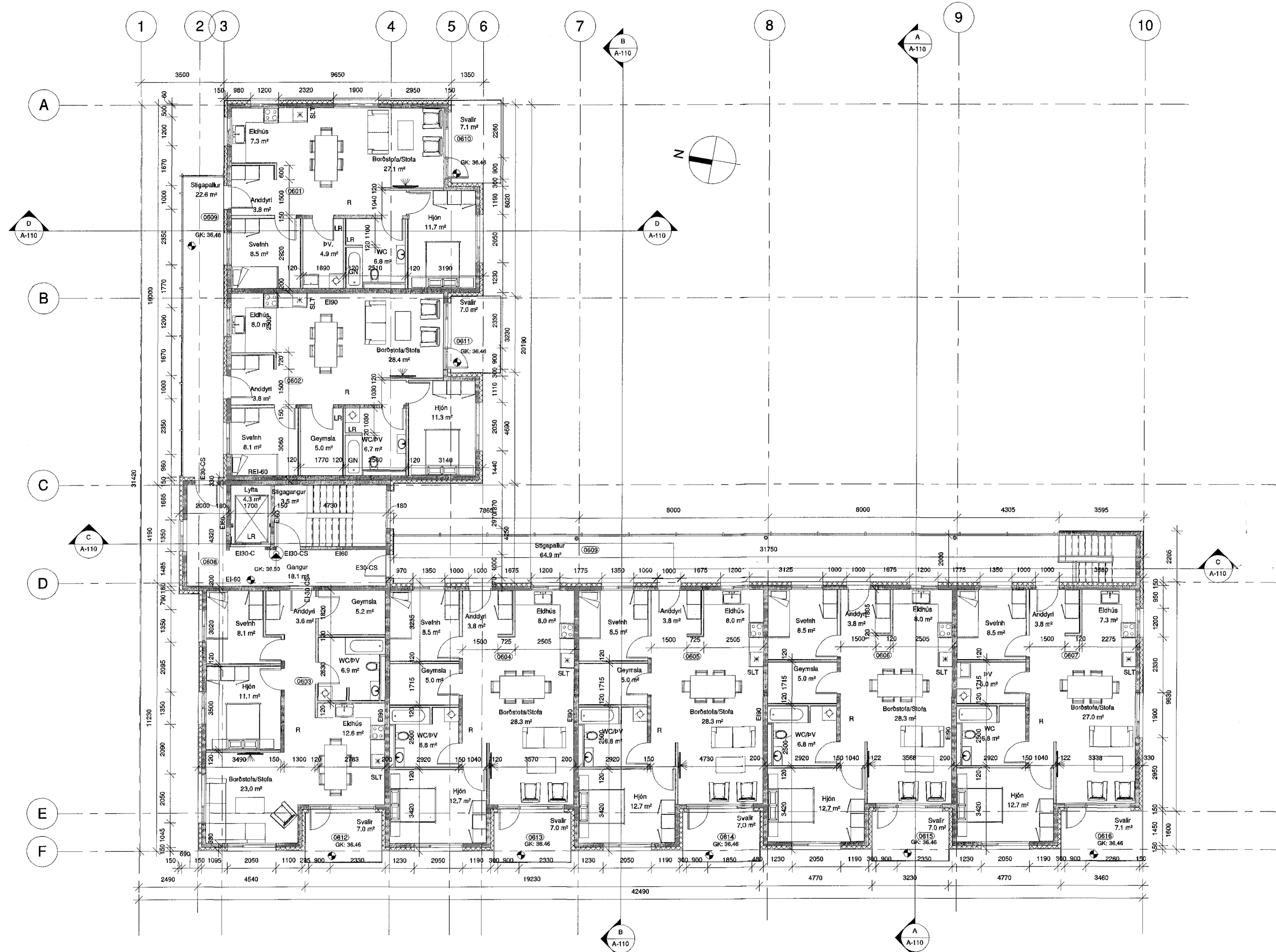
1 6. Hæð 1:100
