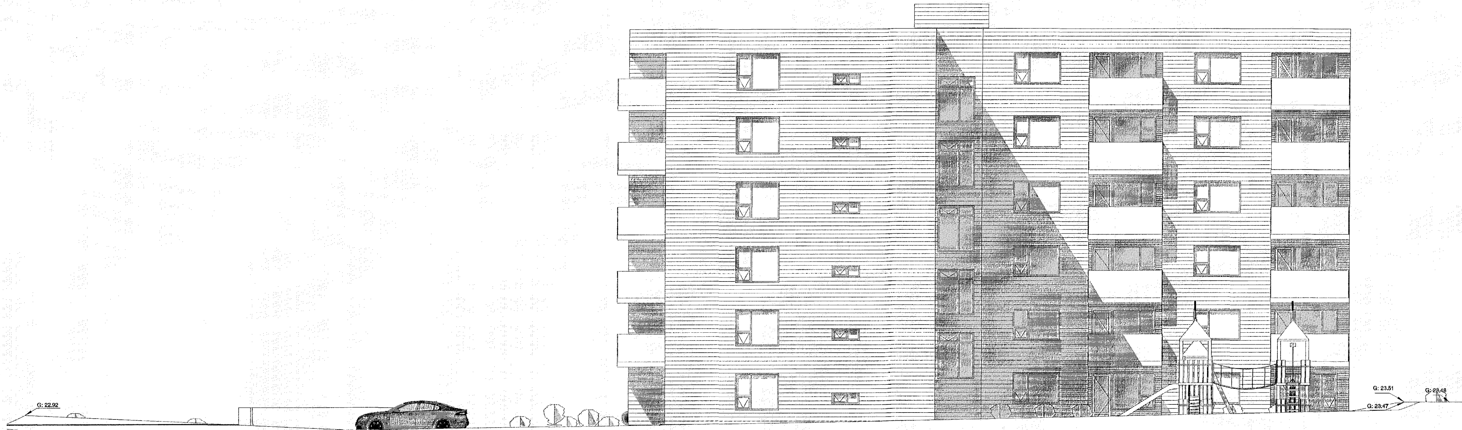
1 Suður 1 : 100
