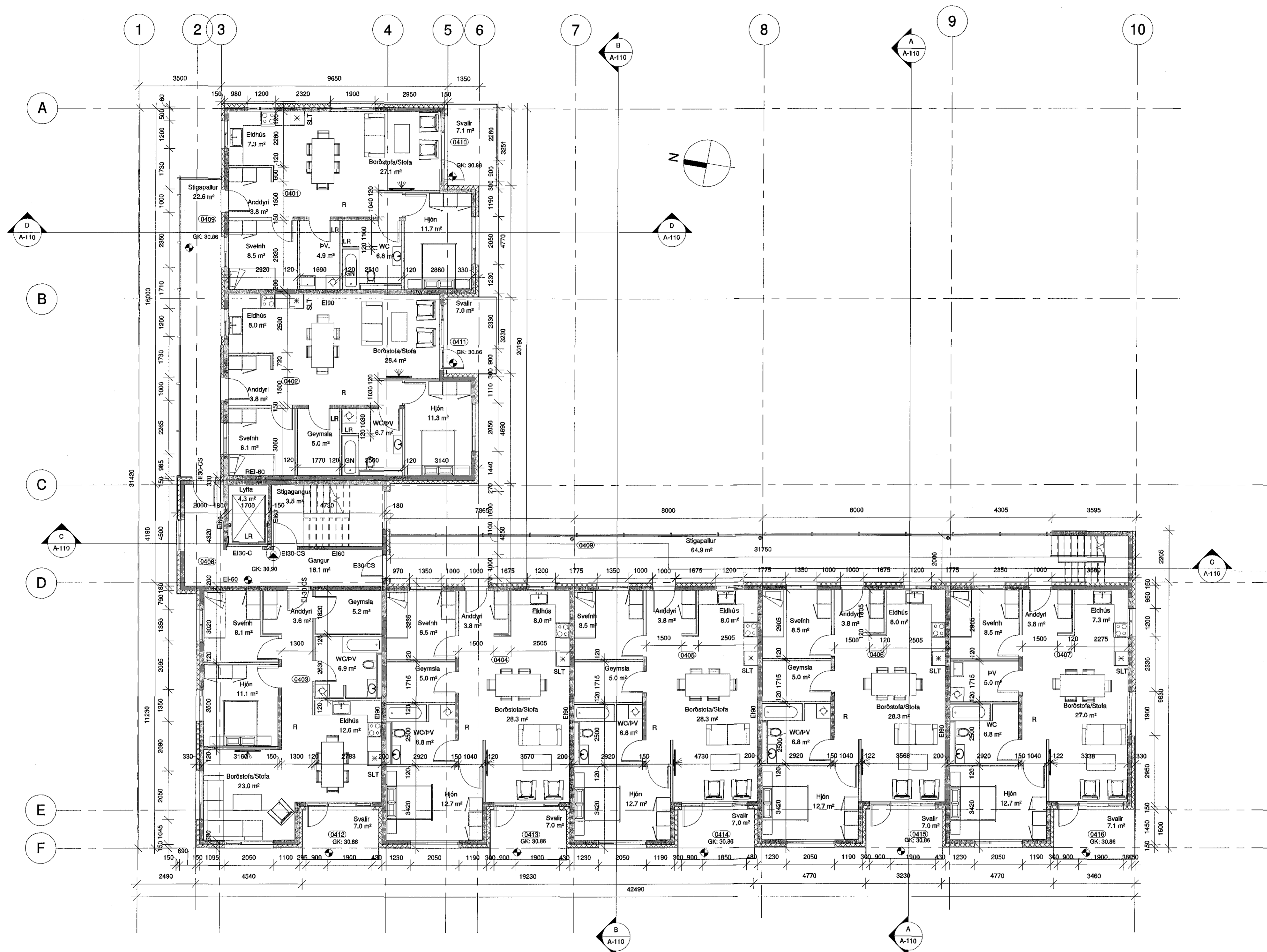
1 4.Hæð 1 : 100
