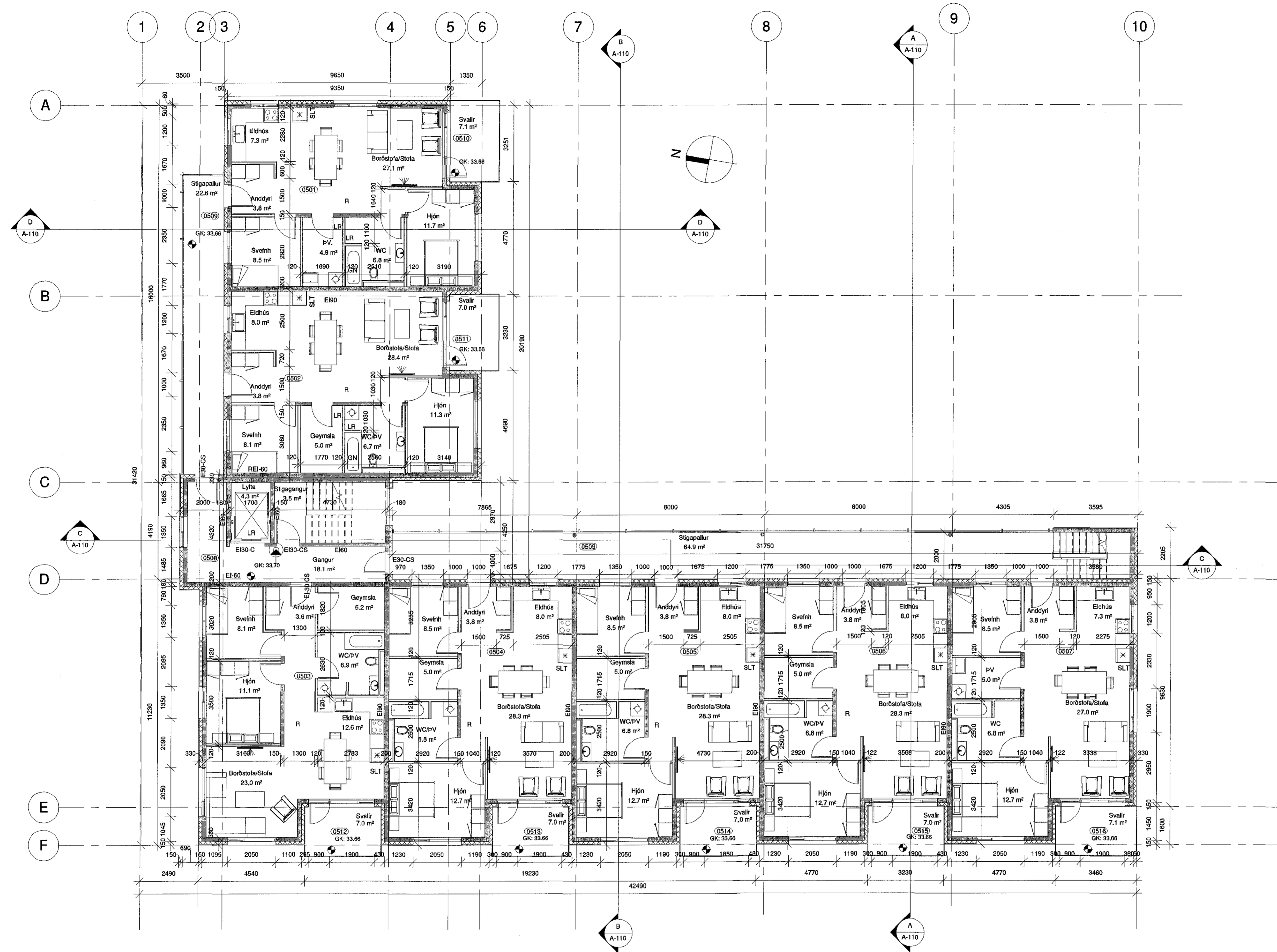
1 5. hæð 1 : 100
