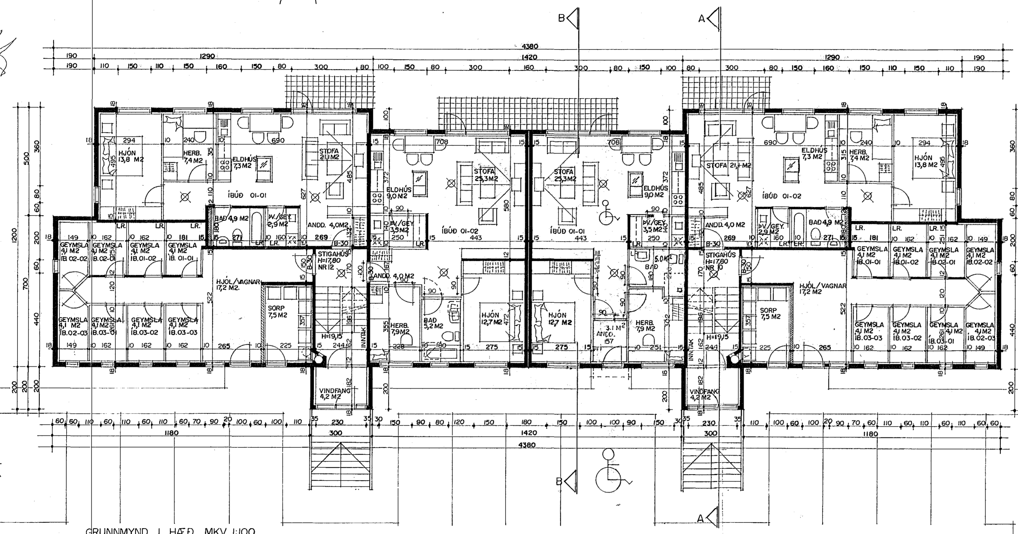
GRUNNMYND I HÆÐ MKV. 1:100
