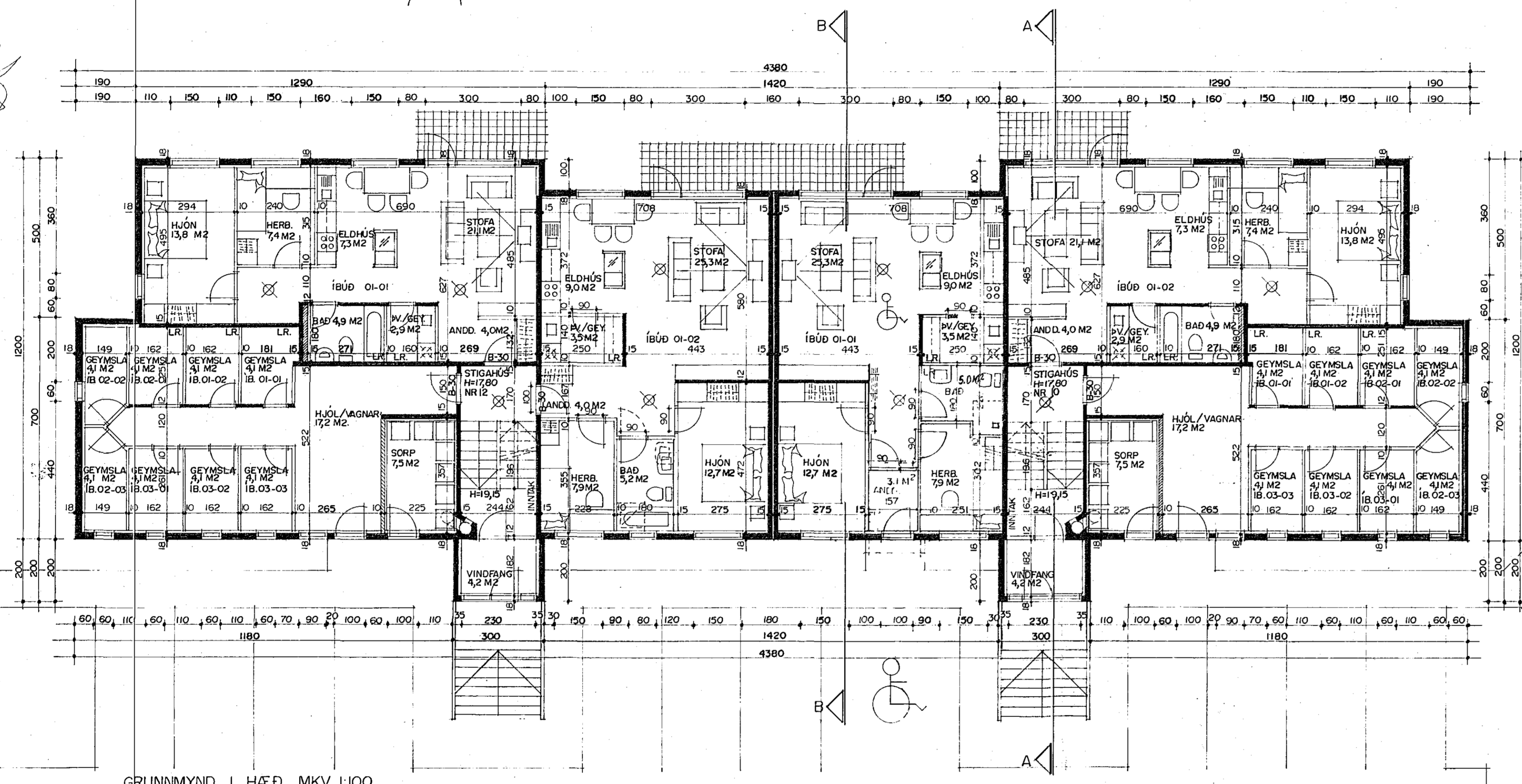
GRUNNMYND I HÆÐ MKV. 1:100
