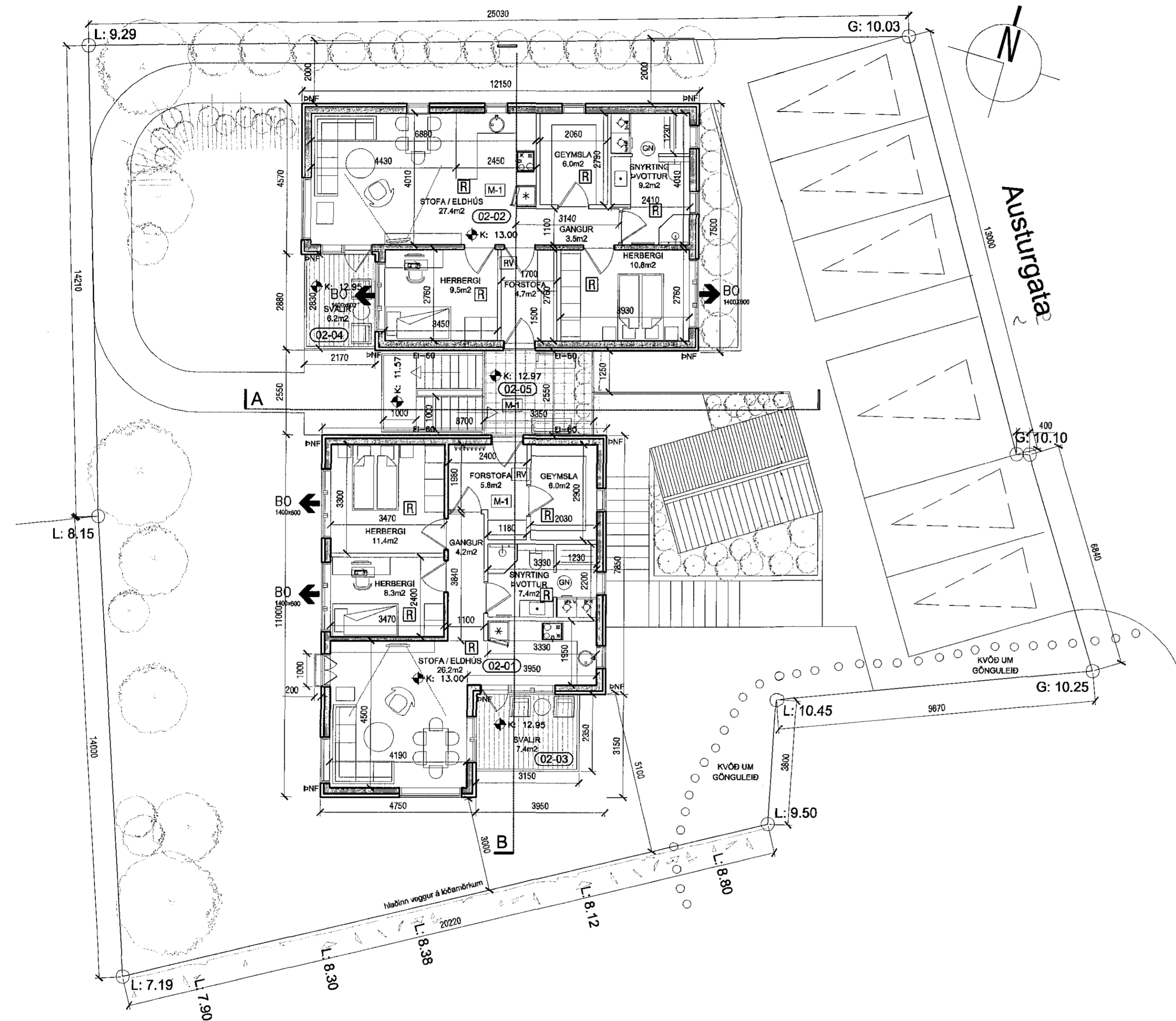
Grunnmynd - 3.hæð mkv. 1:100
