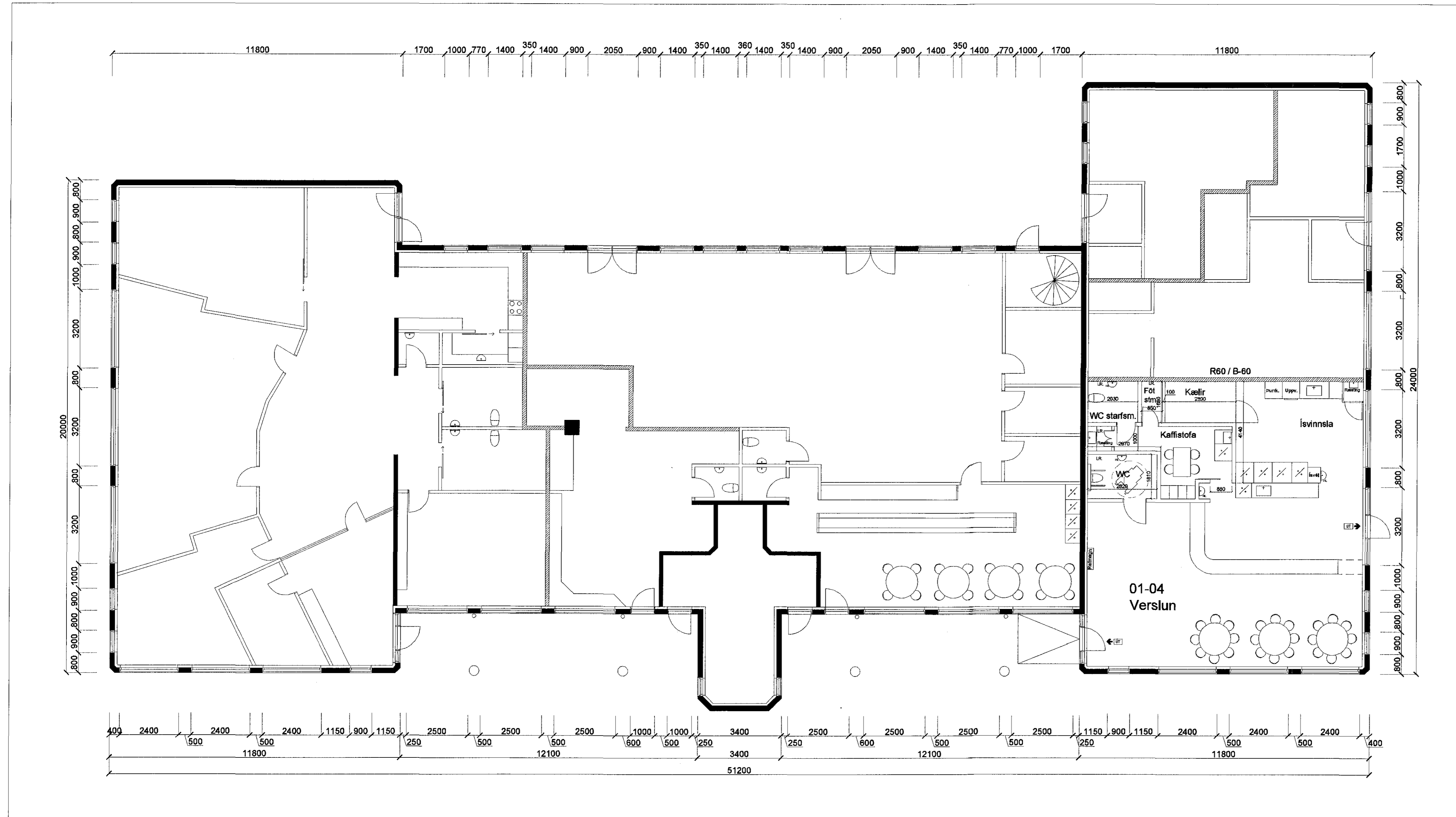
Grunnmynd 1.h. mkv 1:100
