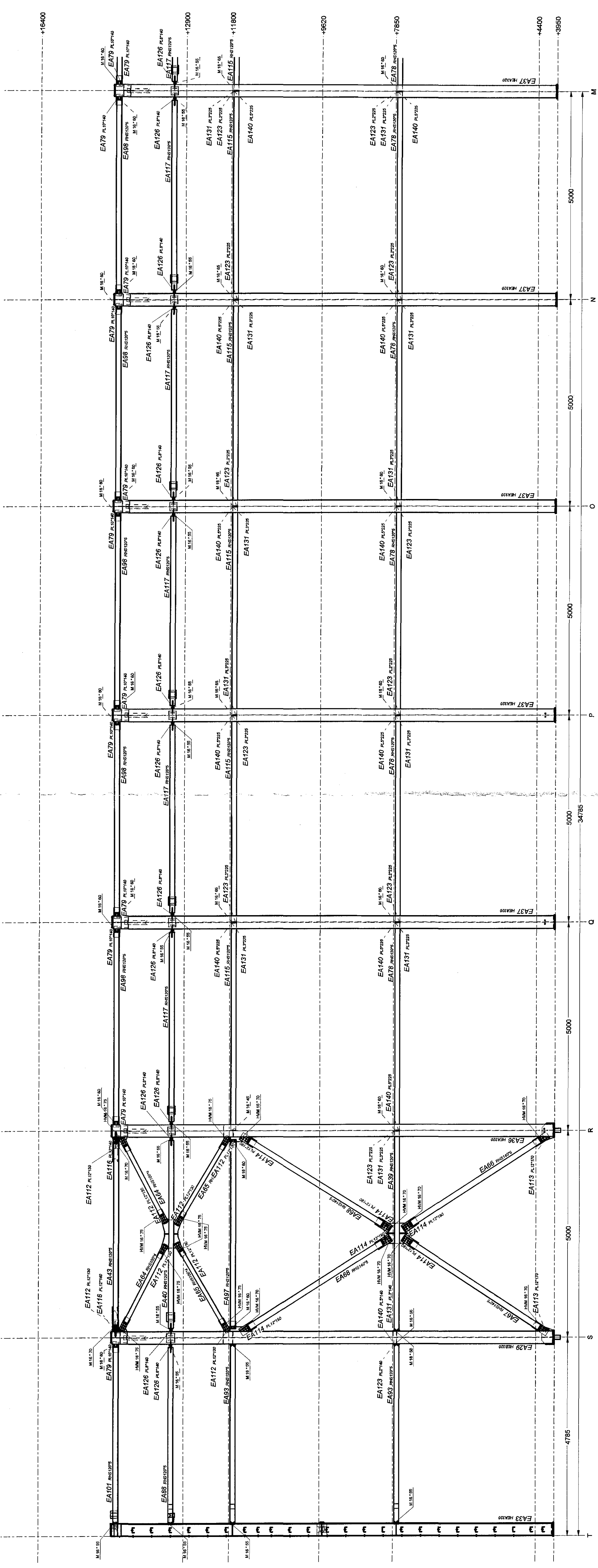
AXIS 17 1:50
