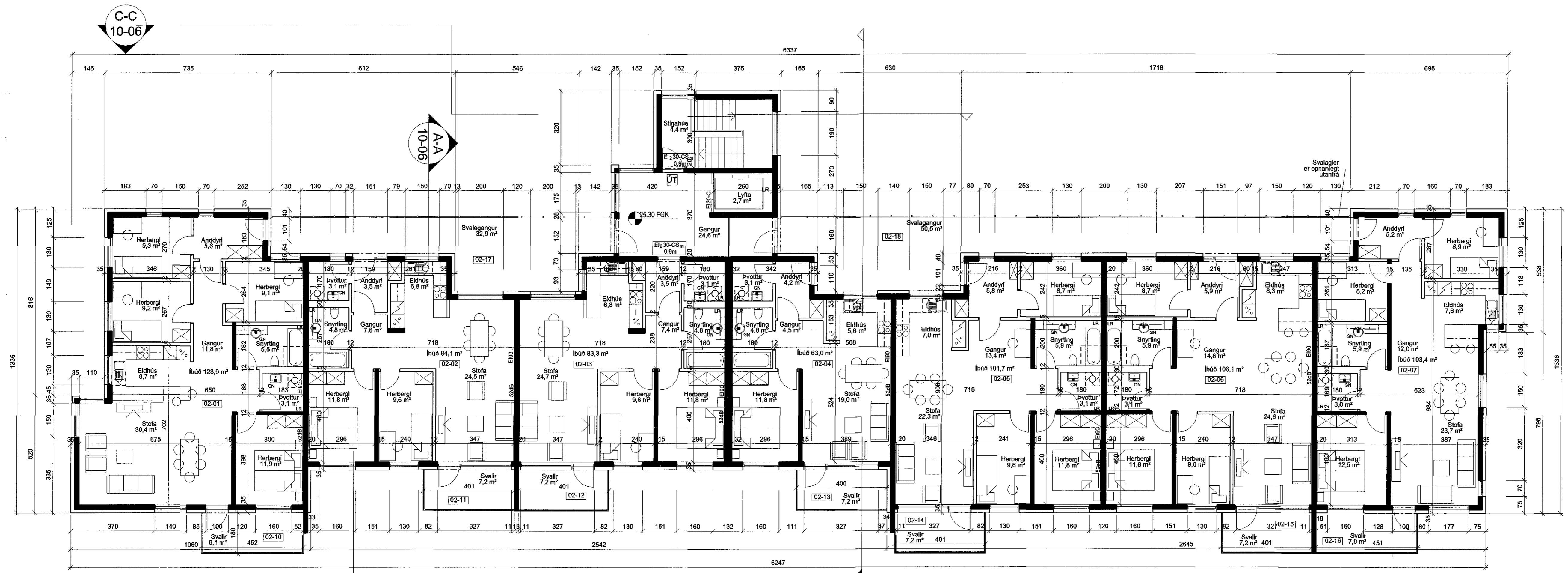
GRUNNMYND 1:100 2. HÆÐ
