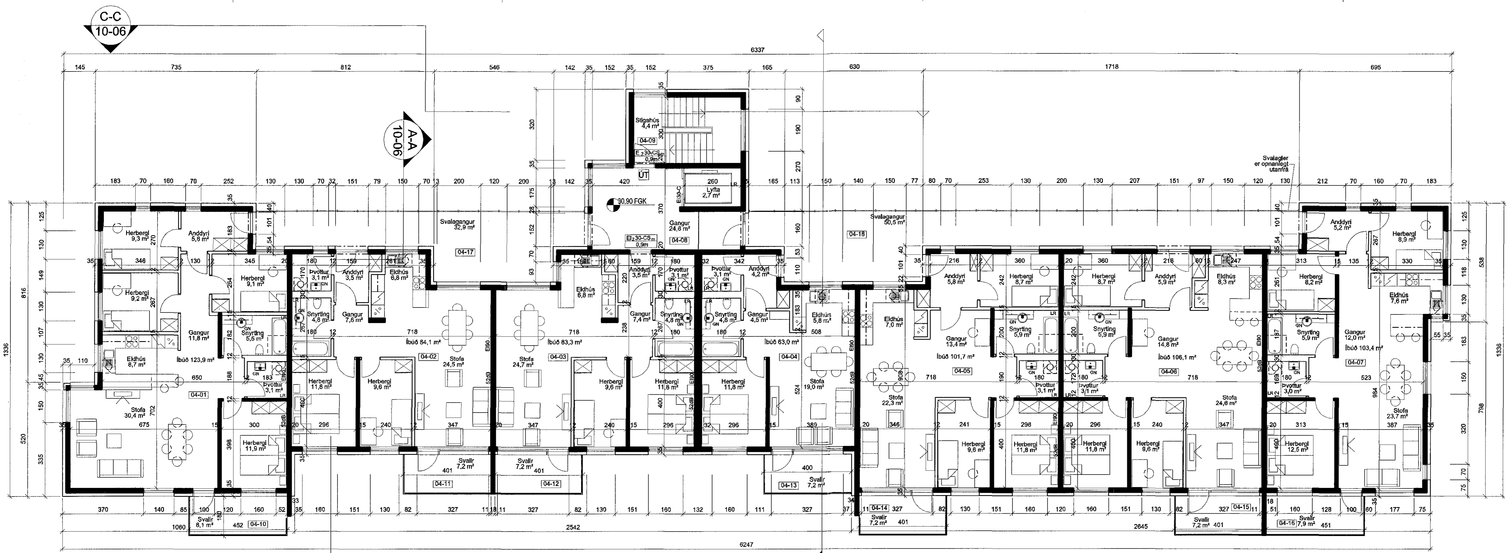
GRUNNMYND 1:100 4. HÆÐ
