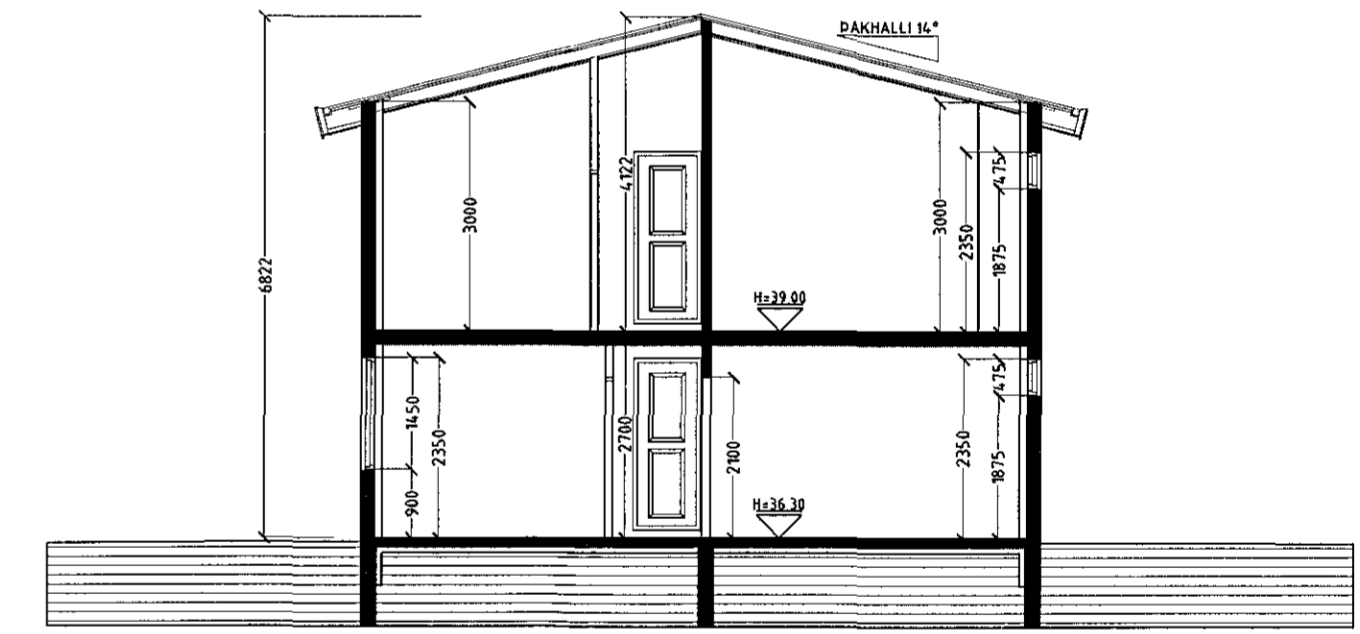
SNÍÐ B-B MKV. 1:100.
