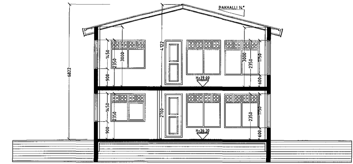
SNÍÐ A-A MKV. 1:100.
