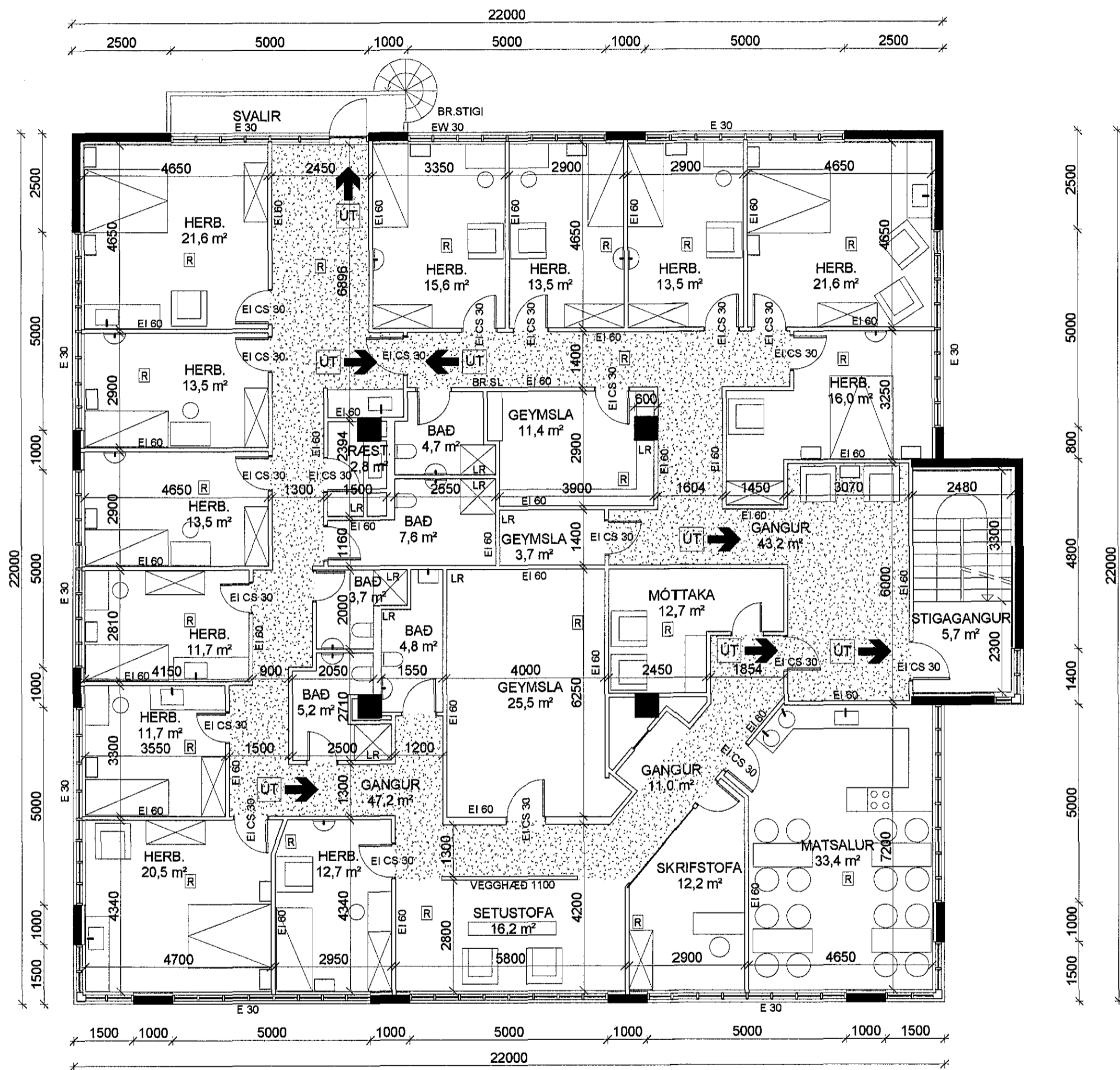
1 GRUNNMYND 2. hæð 1:100
