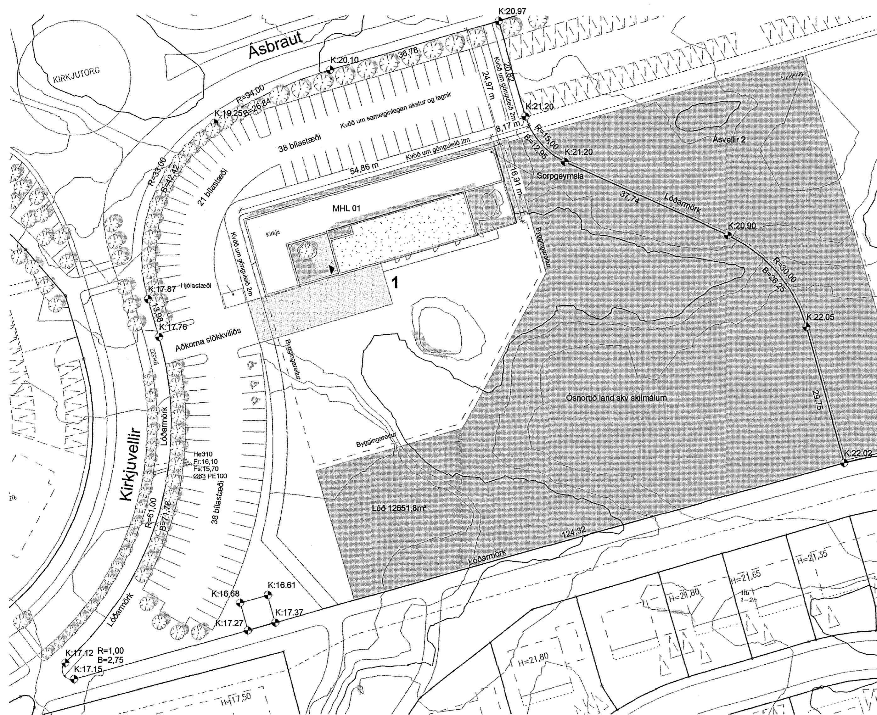
1 Afstöðumynd 1 : 500
