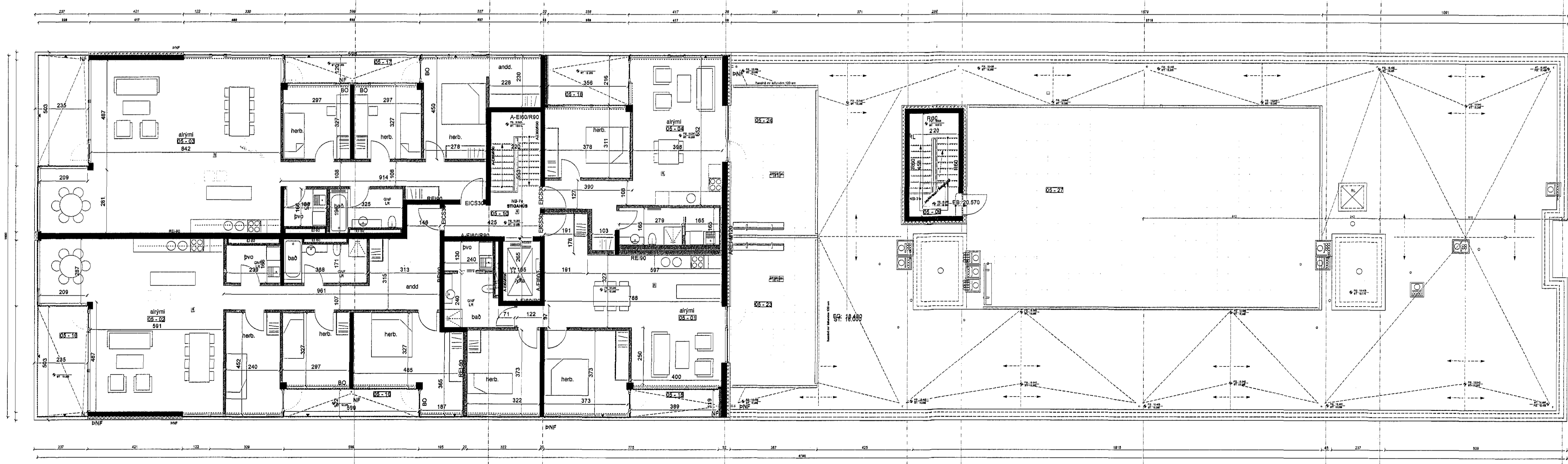
Norðurbakki 7 5. hæð 1:100
