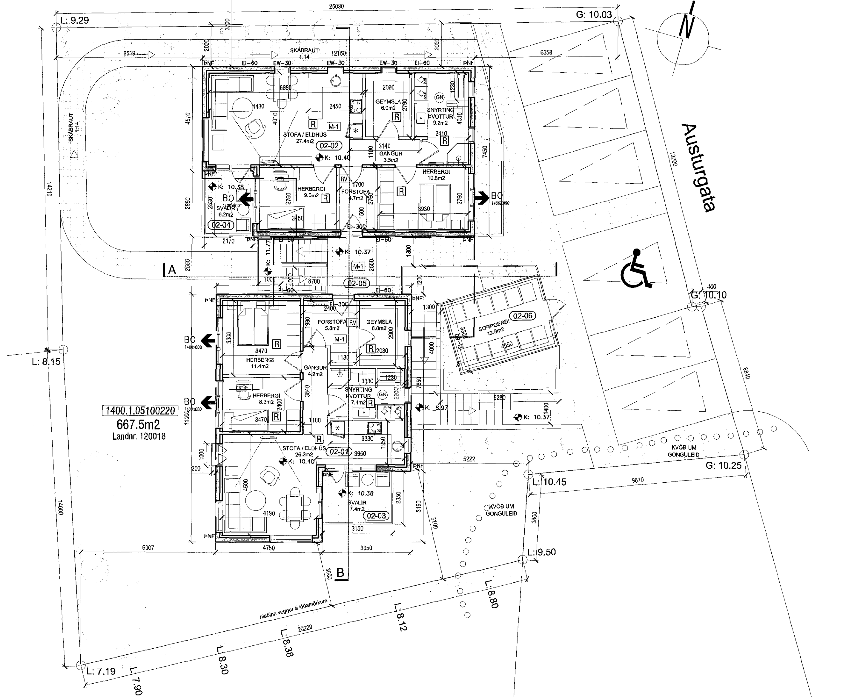
Grunnmynd - 2.hæð mkv. 1:100
