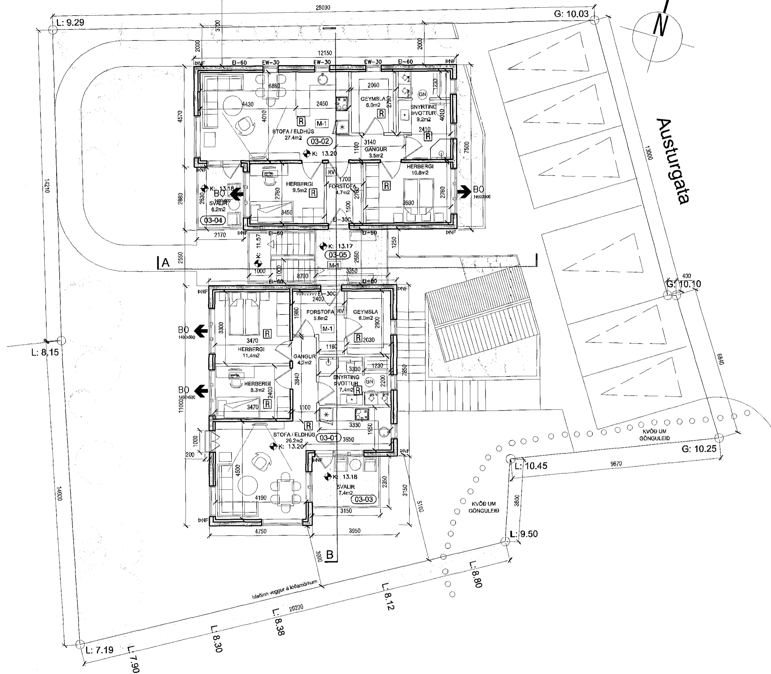
Grunnmynd - 3.hæð mkv. 1:100
