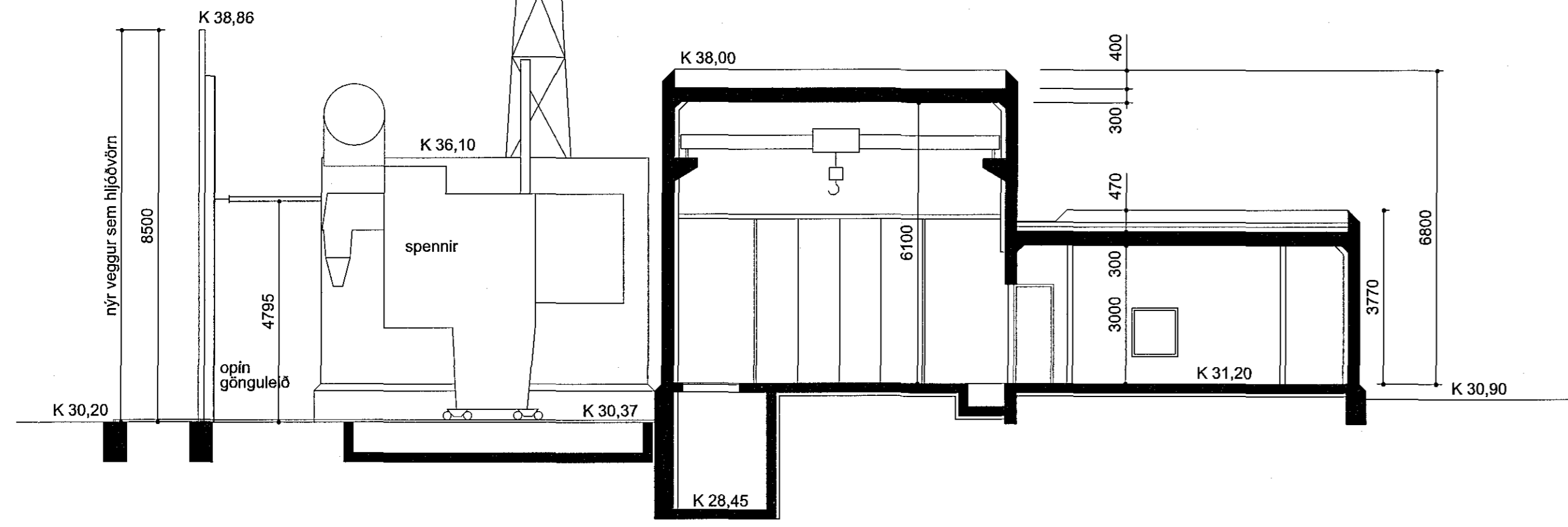
SKURÐMYND A-A 1:100
