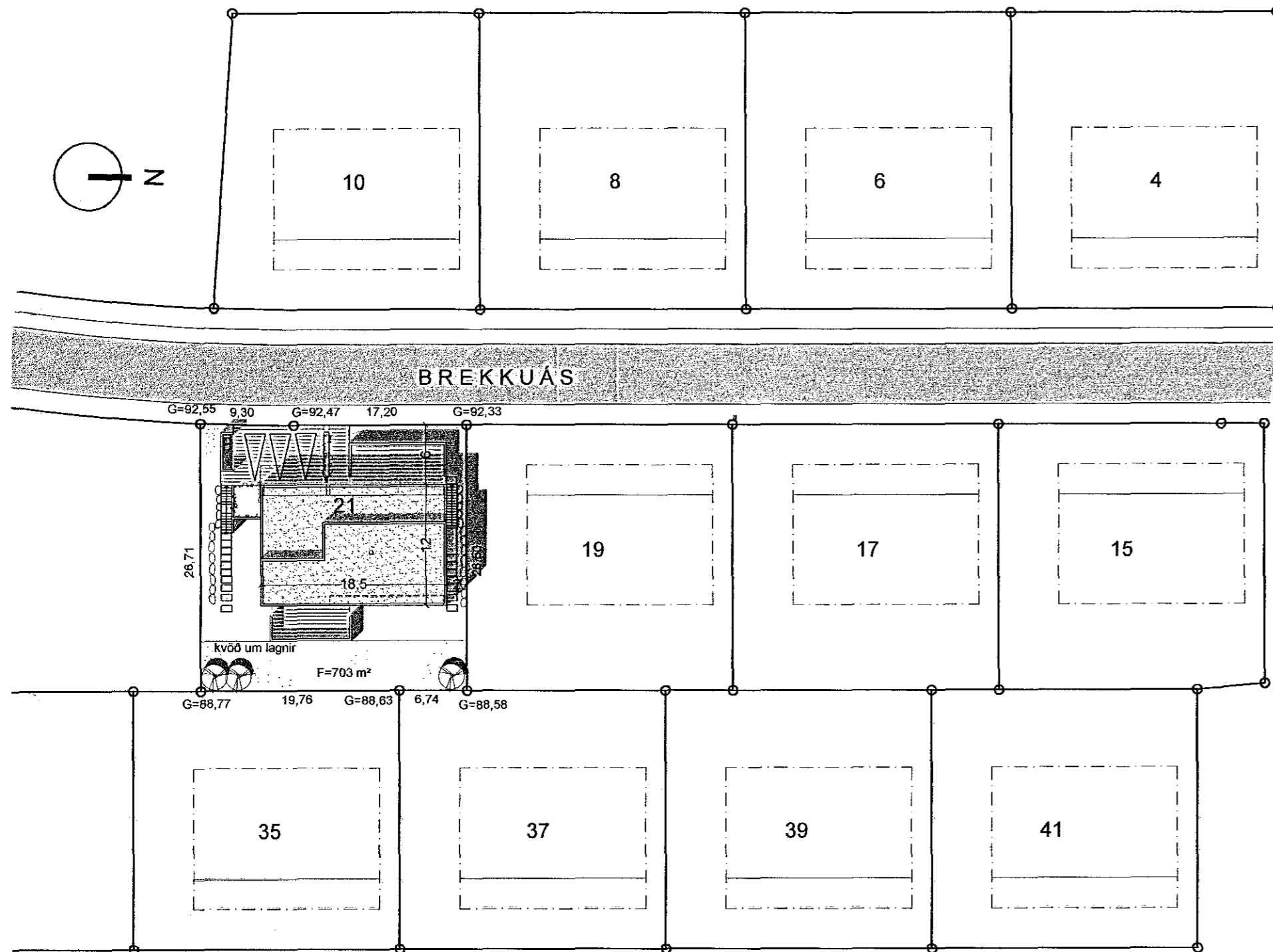
AFSTÖÐUMYND M 1 : 500
