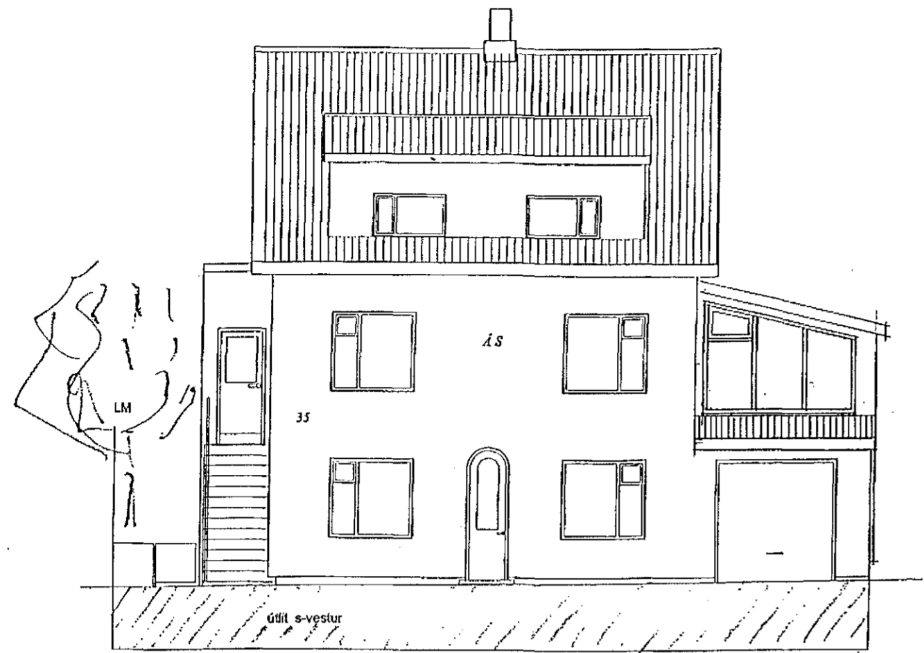
1:100 Útlit, suður-vestur
