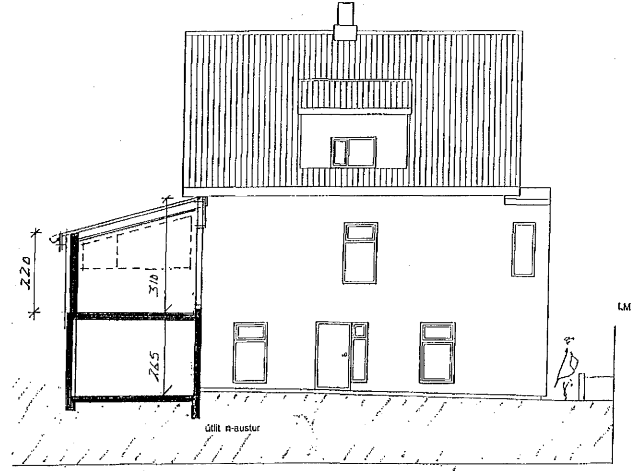
1:100 Útlit, norður-austur
