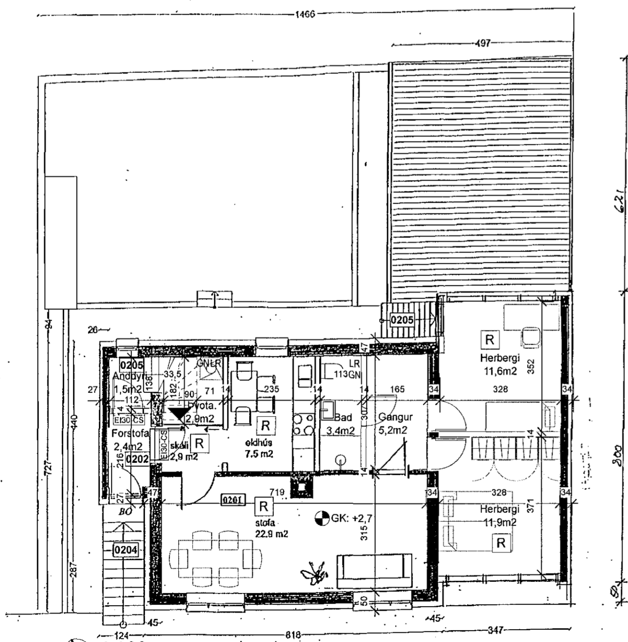
1:100 Grunnmynd, 2.hæð
