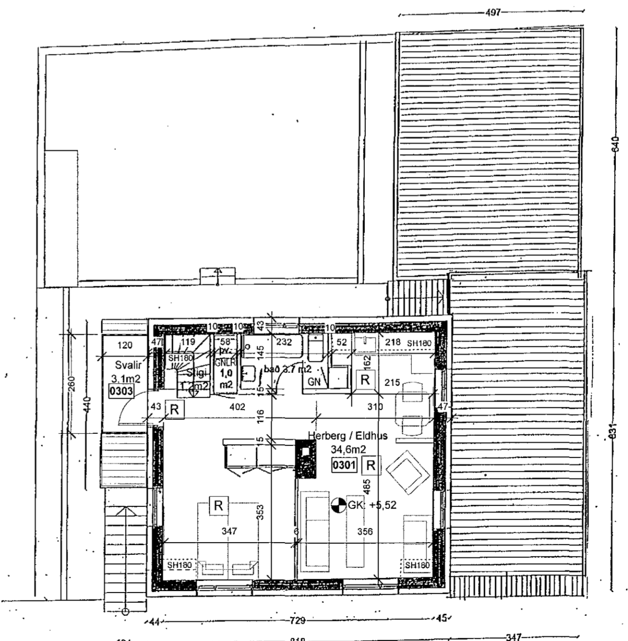
1:100 Grunnmynd, 3.hæð
