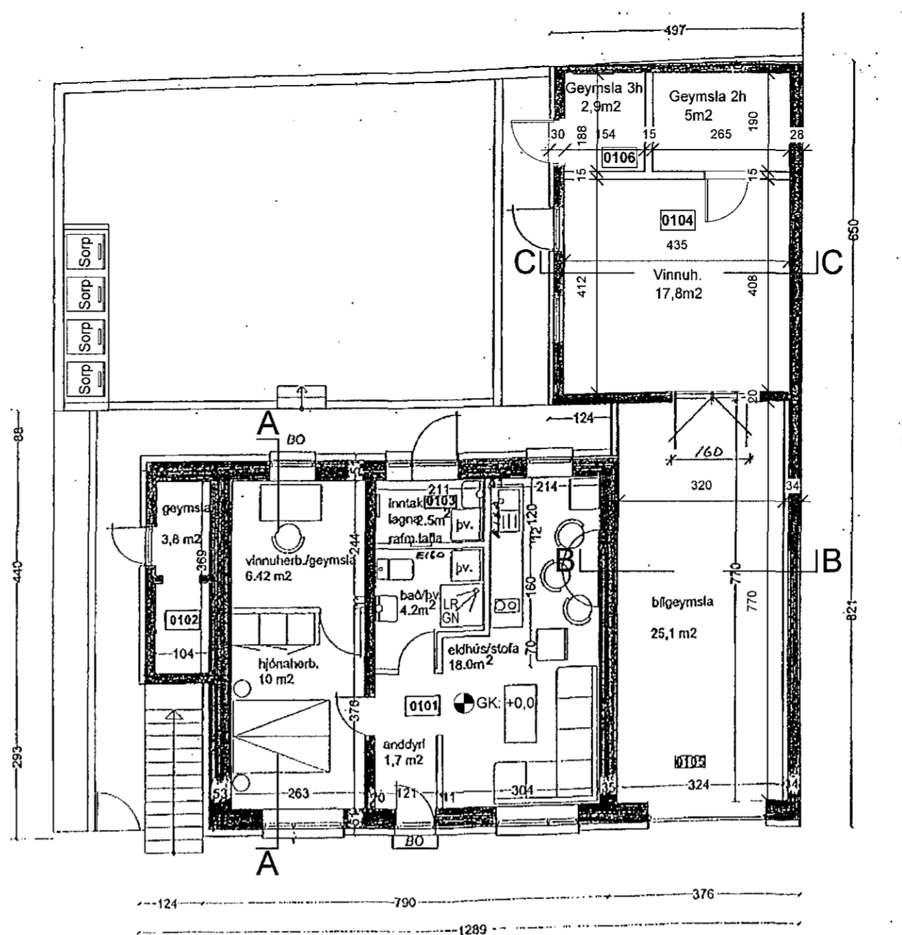
1:100 Grunnmynd, 1.hæð
