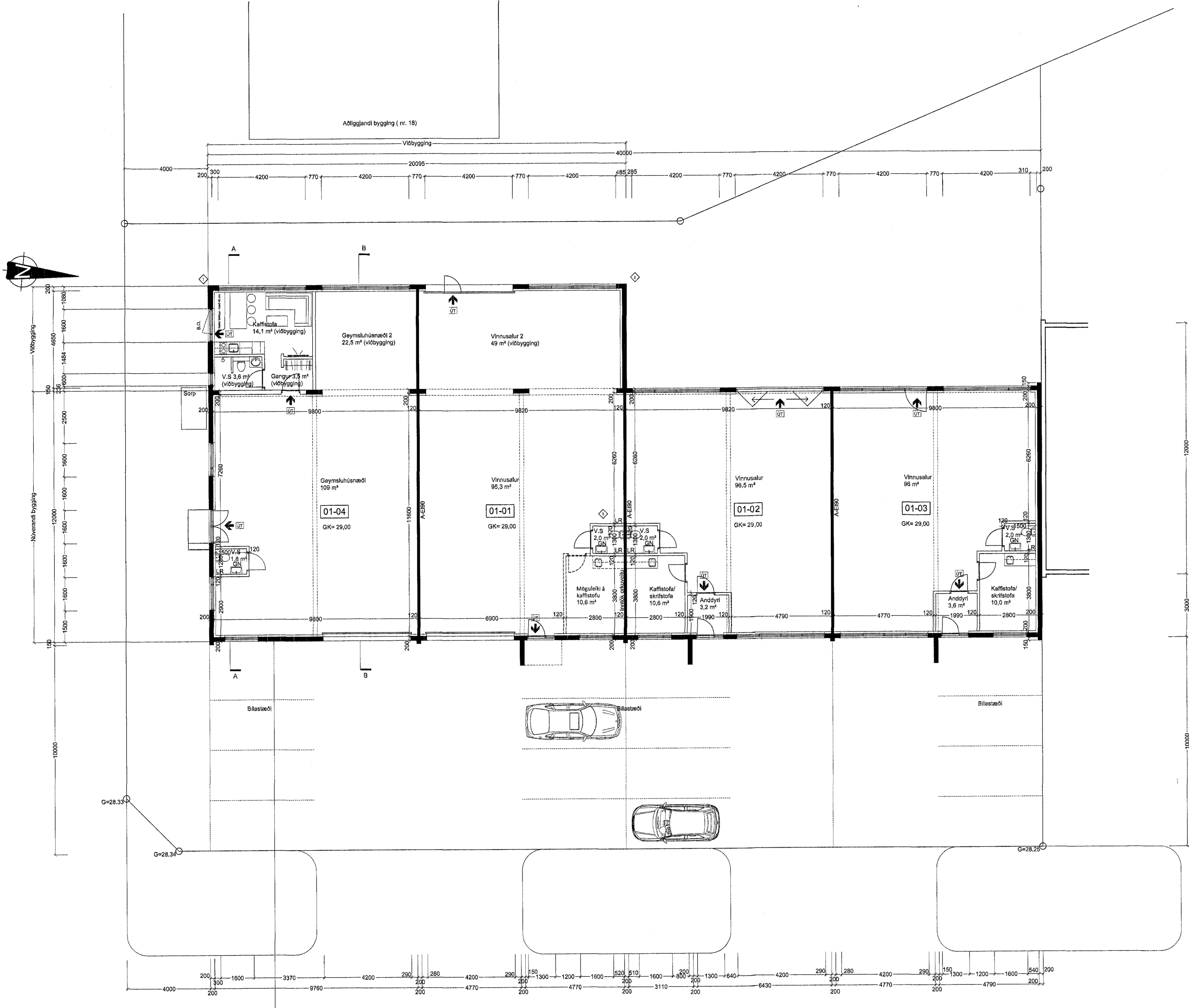
Grunnmynd 1. hæðar 1:100
