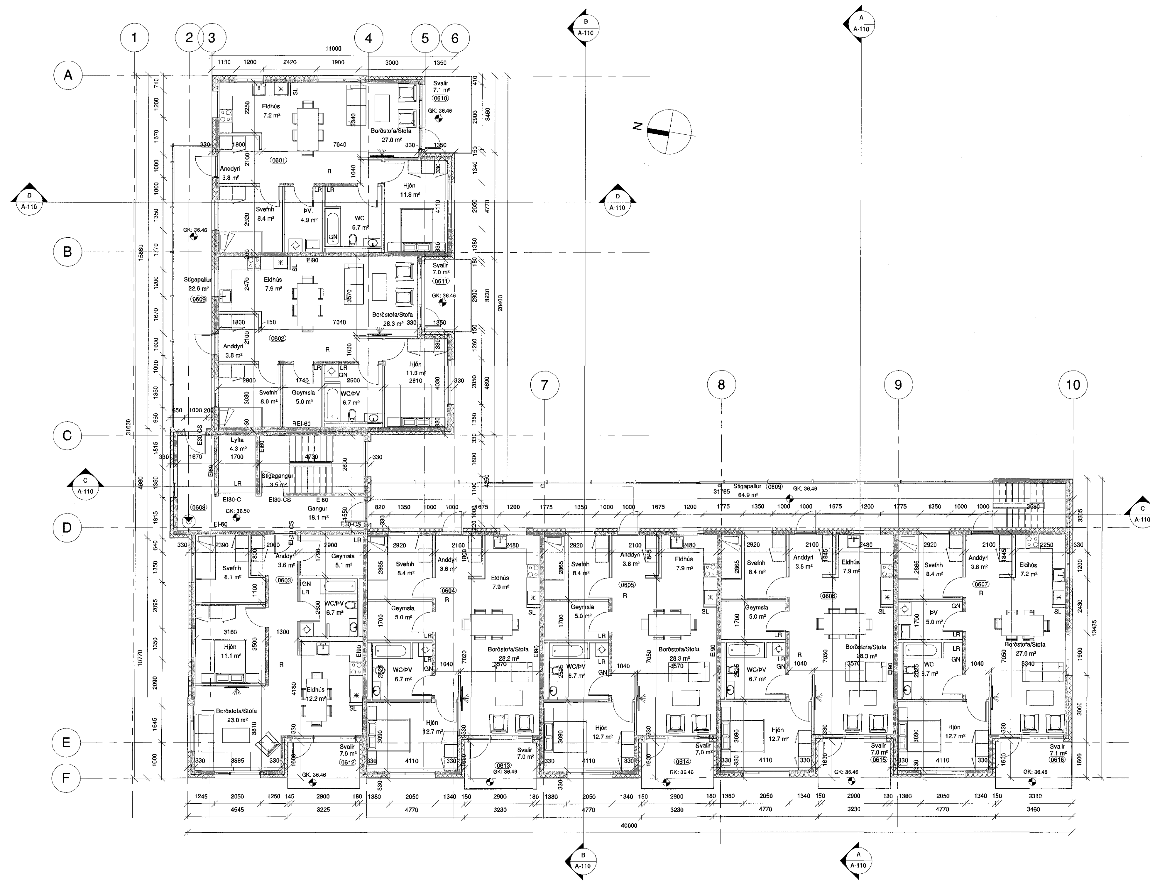
1 6.Hæð 1 : 100
