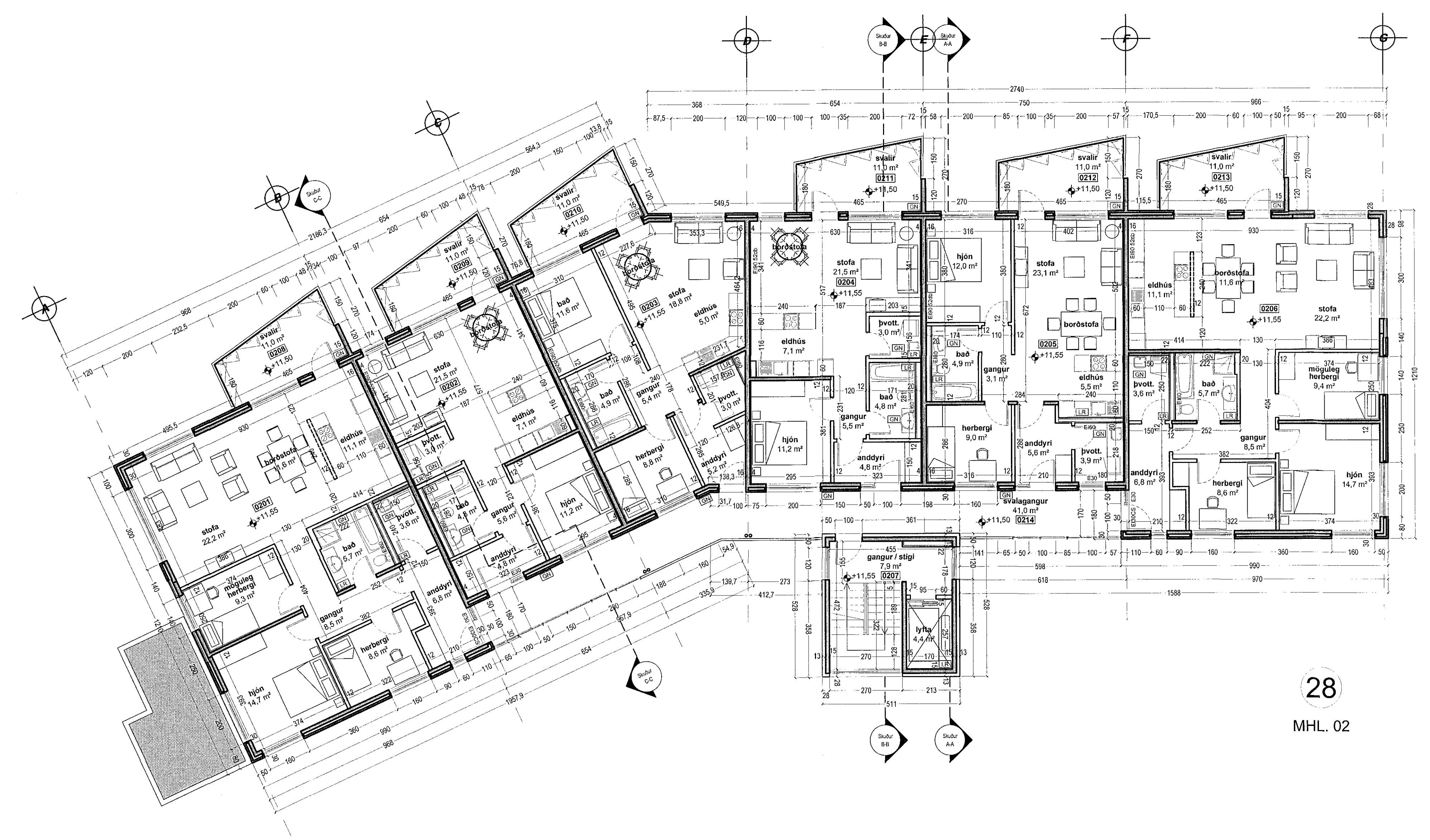
grunnmynd 2.hæð
