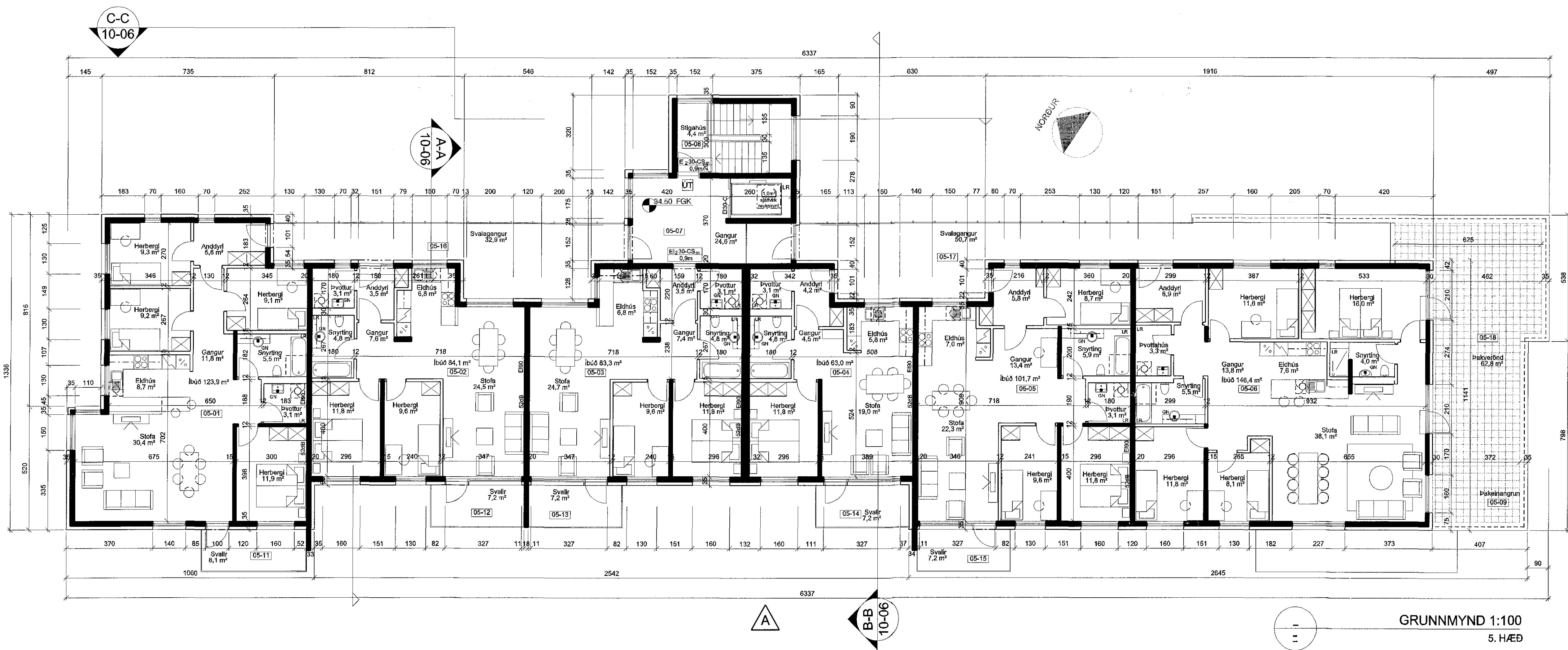
GRUNNMYND 1:100 4. HÆÐ
