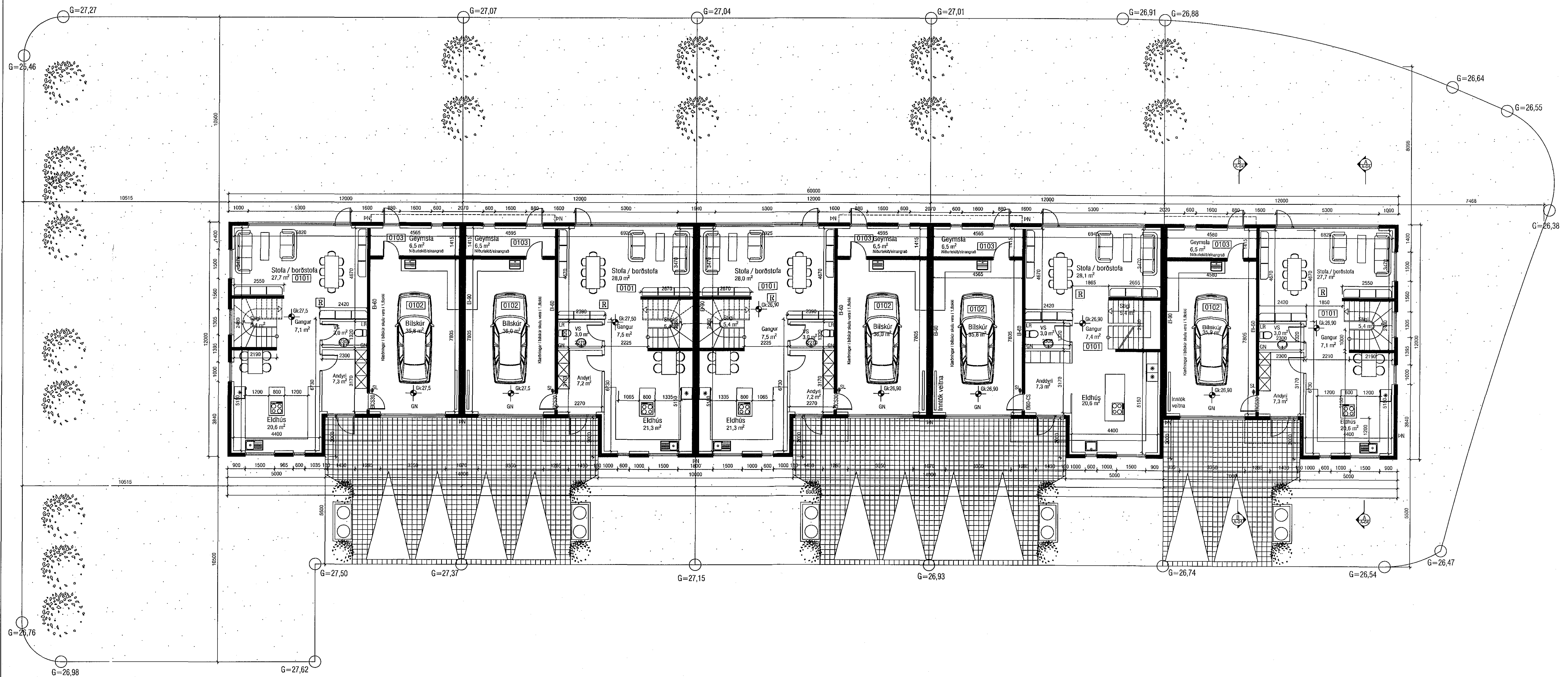
GRUNNMYND 1.HÆÐ 1:100
