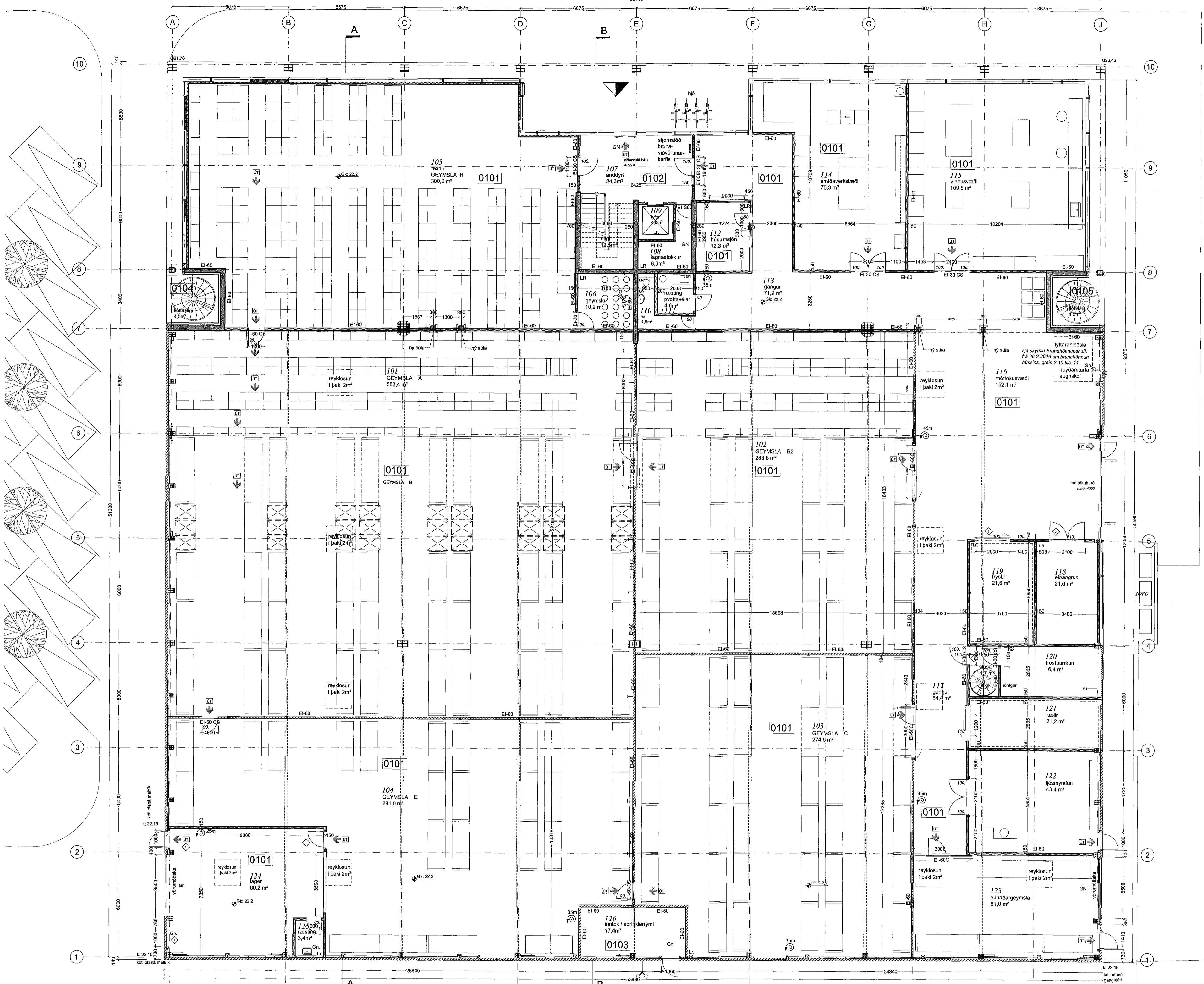
GRUNNMYND 1. HÆÐ M 1 : 100
