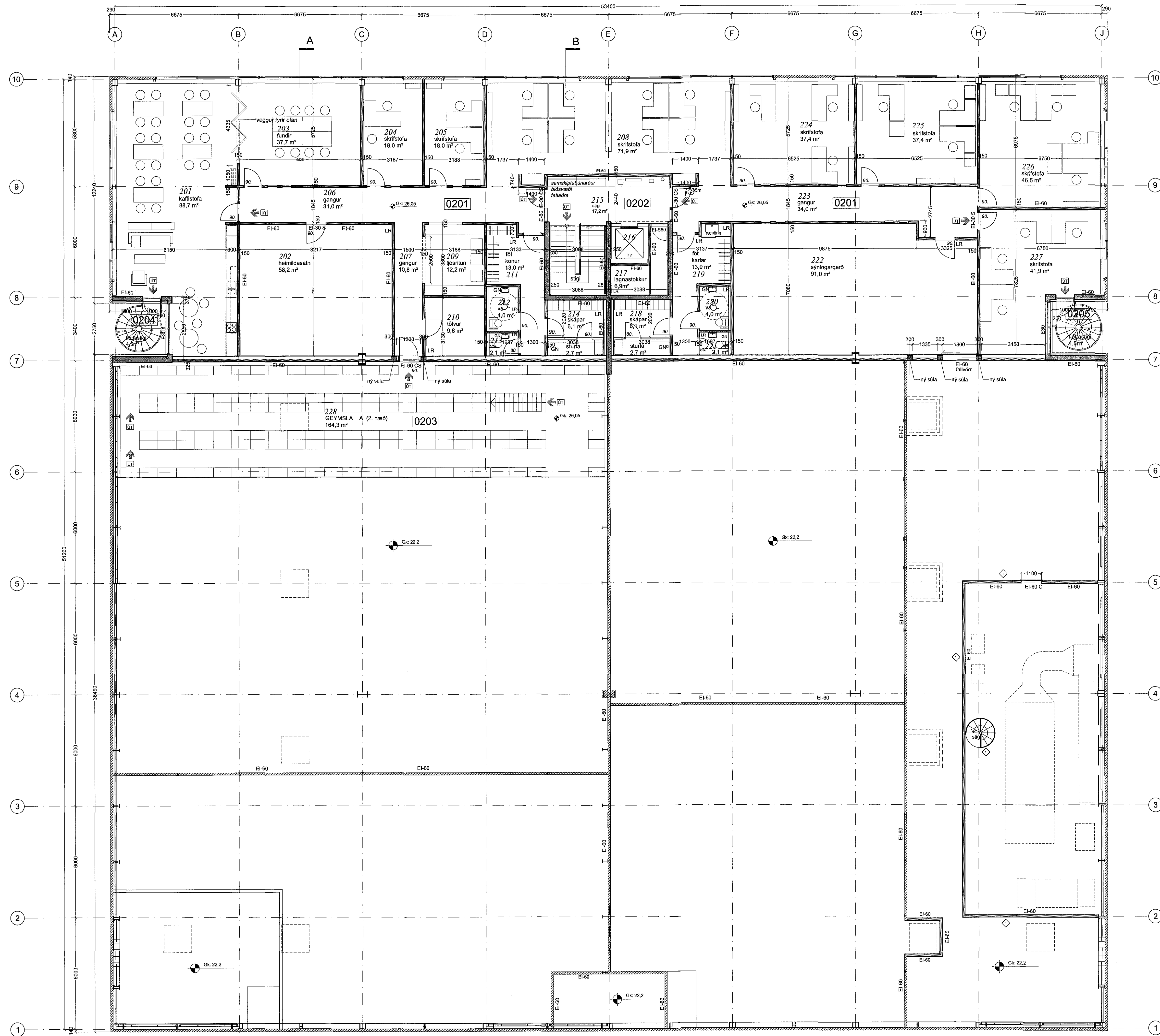
GRUNNMYND 2. HÆÐ M 1 : 100
