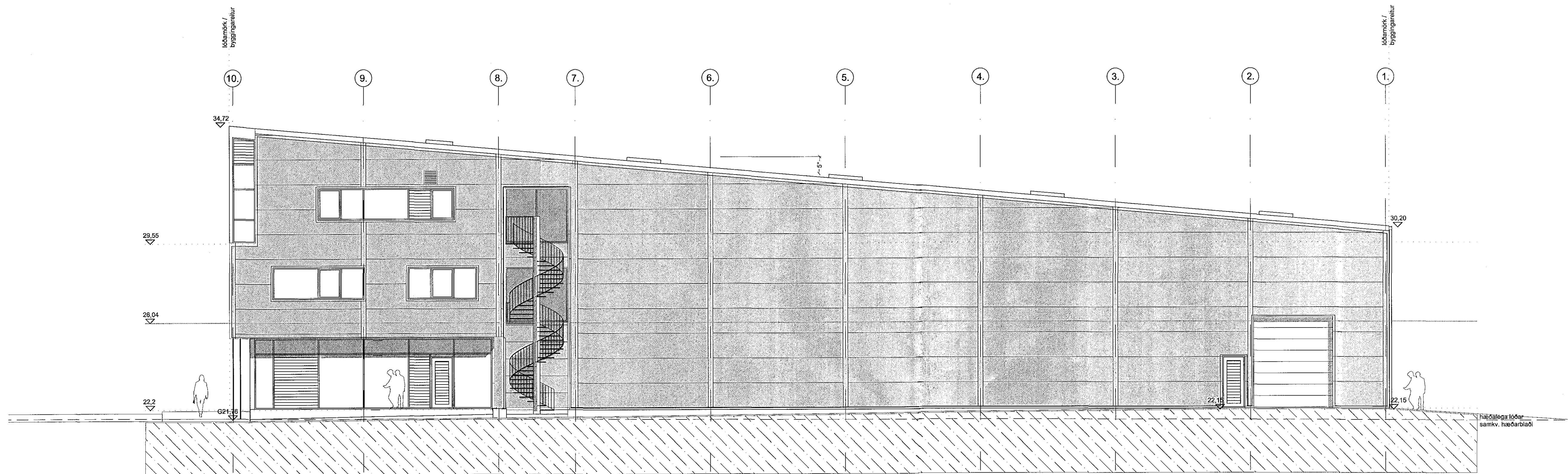
ÚTLIT AUSTUR M 1:100
