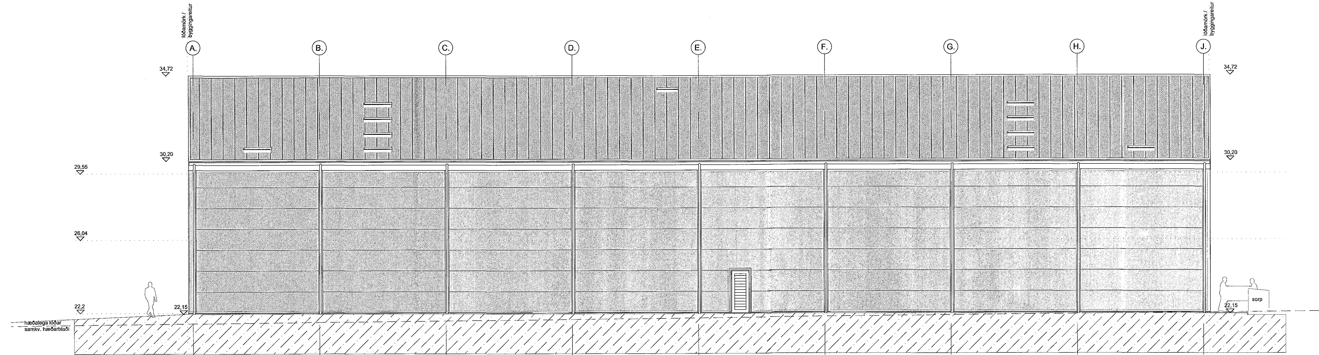
ÚTLIT SUÐUR M 1:100
