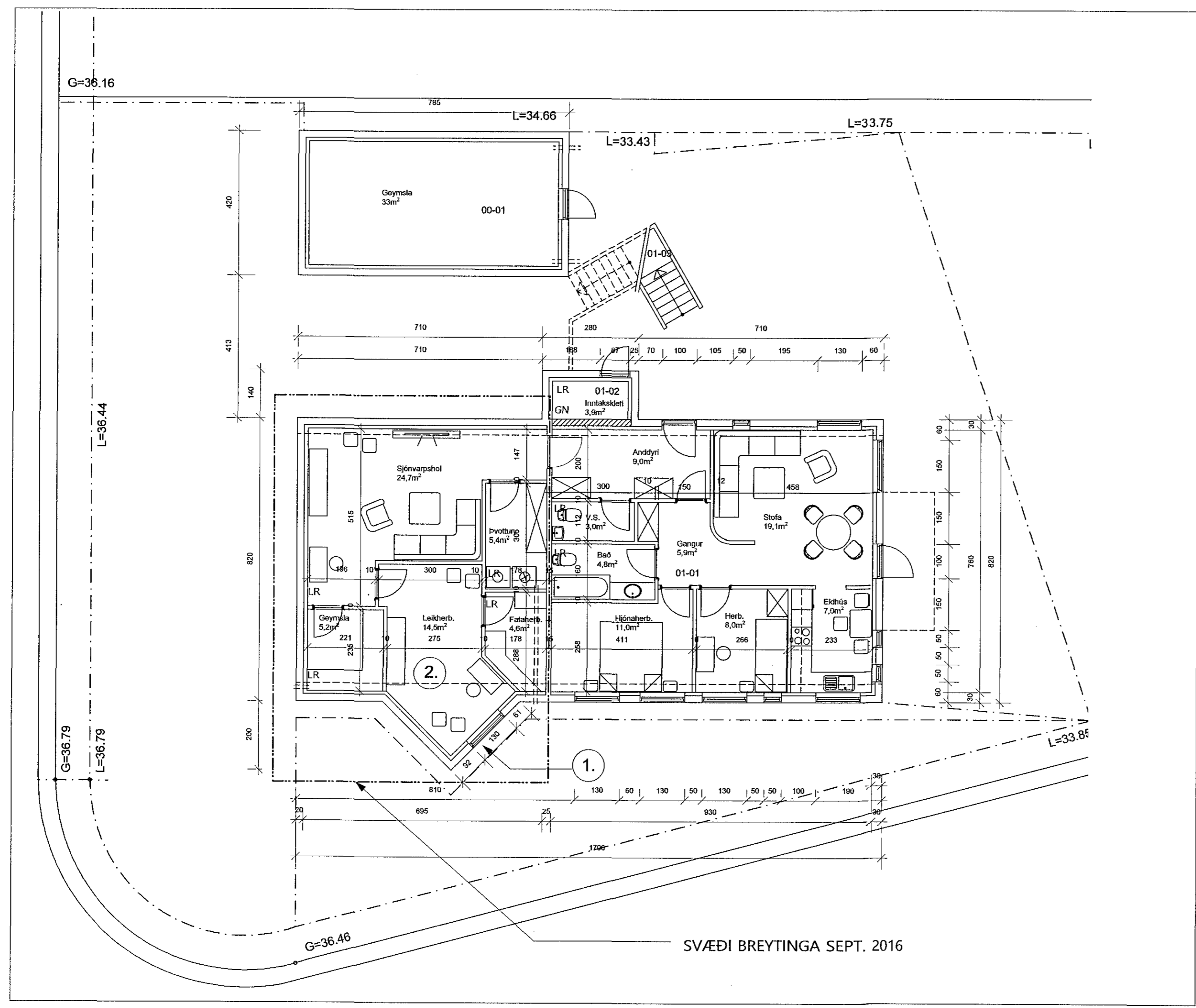
1. hæð 1:100
