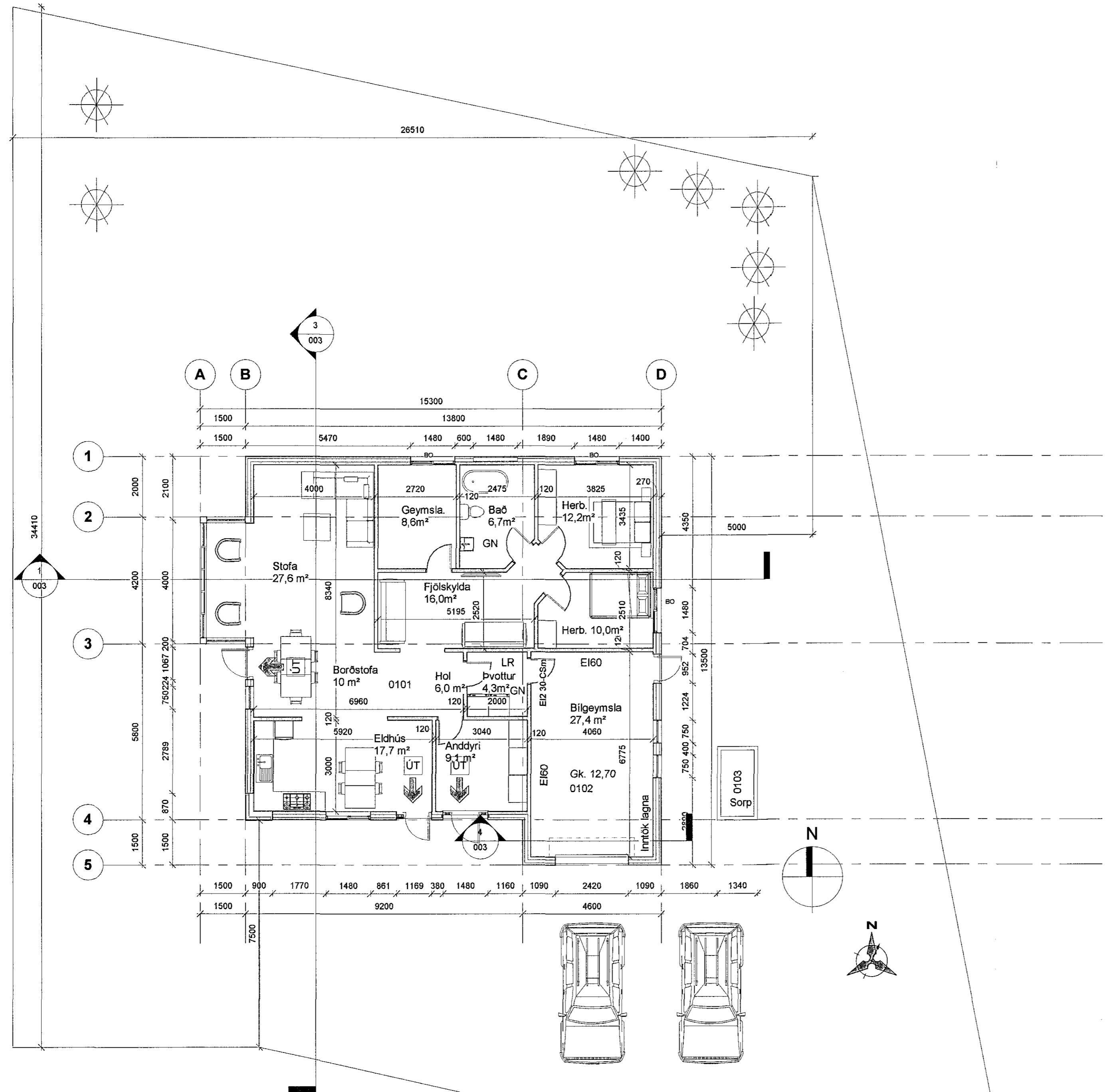
1 01 grunnmynd 1 : 100
