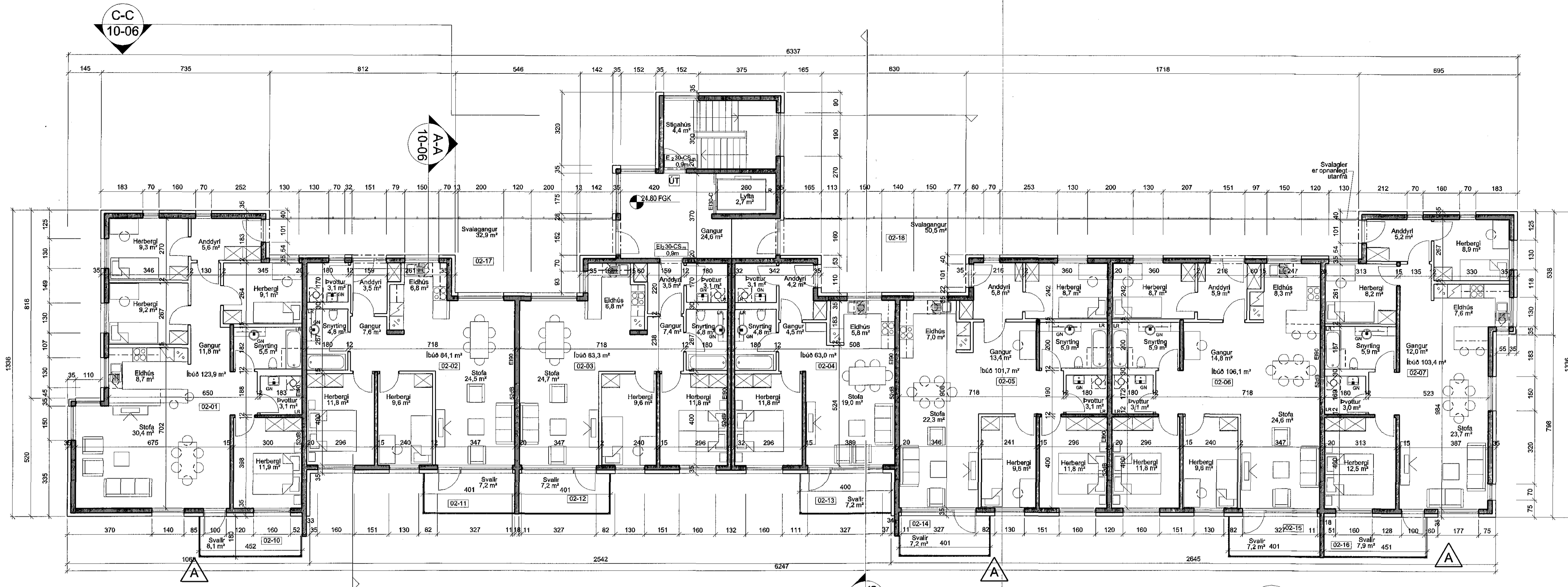
GRUNNMYND 1:100 2. HÆÐ
