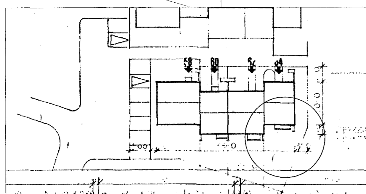
AFSTÖÐUMYND 1:500
