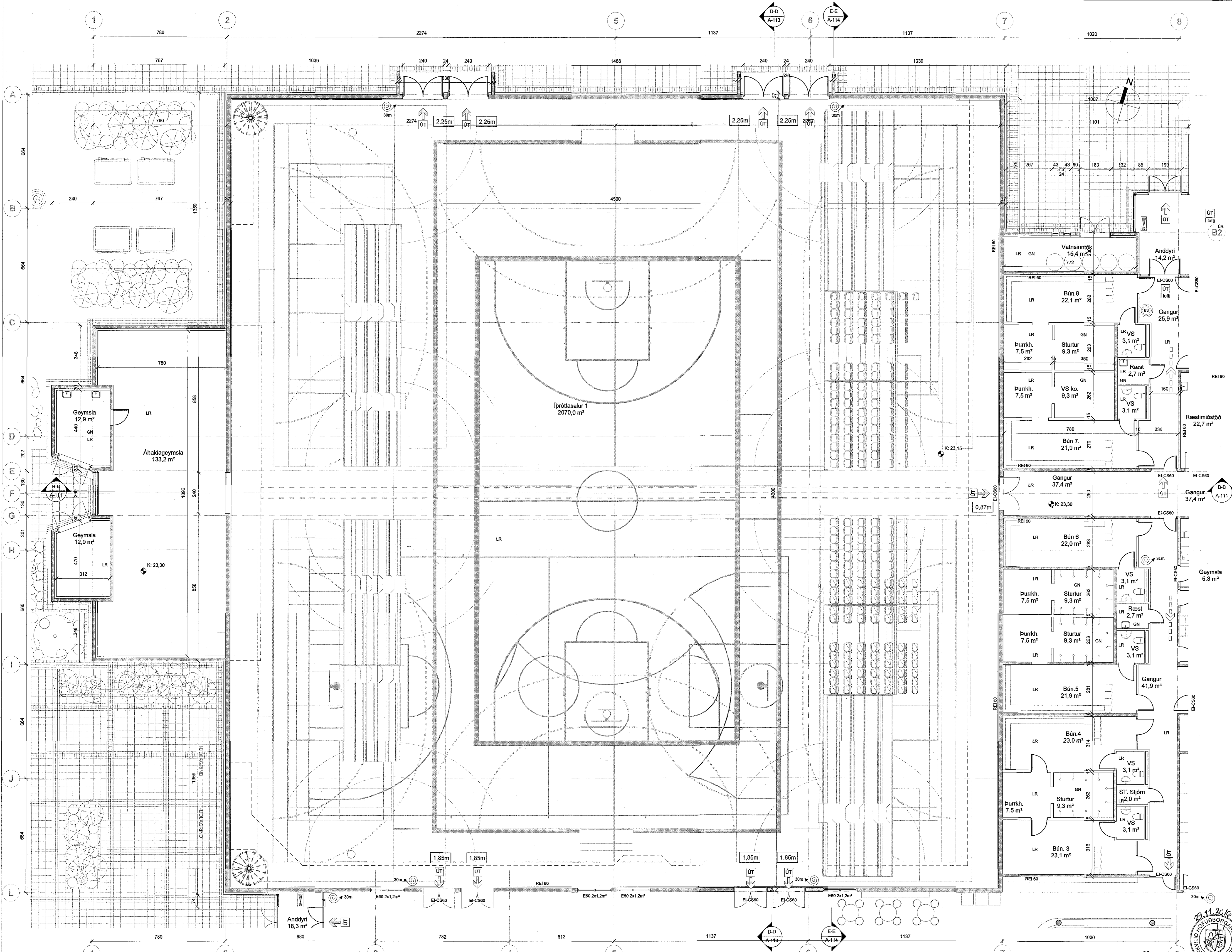
Hæð 1 -N 1 : 100
