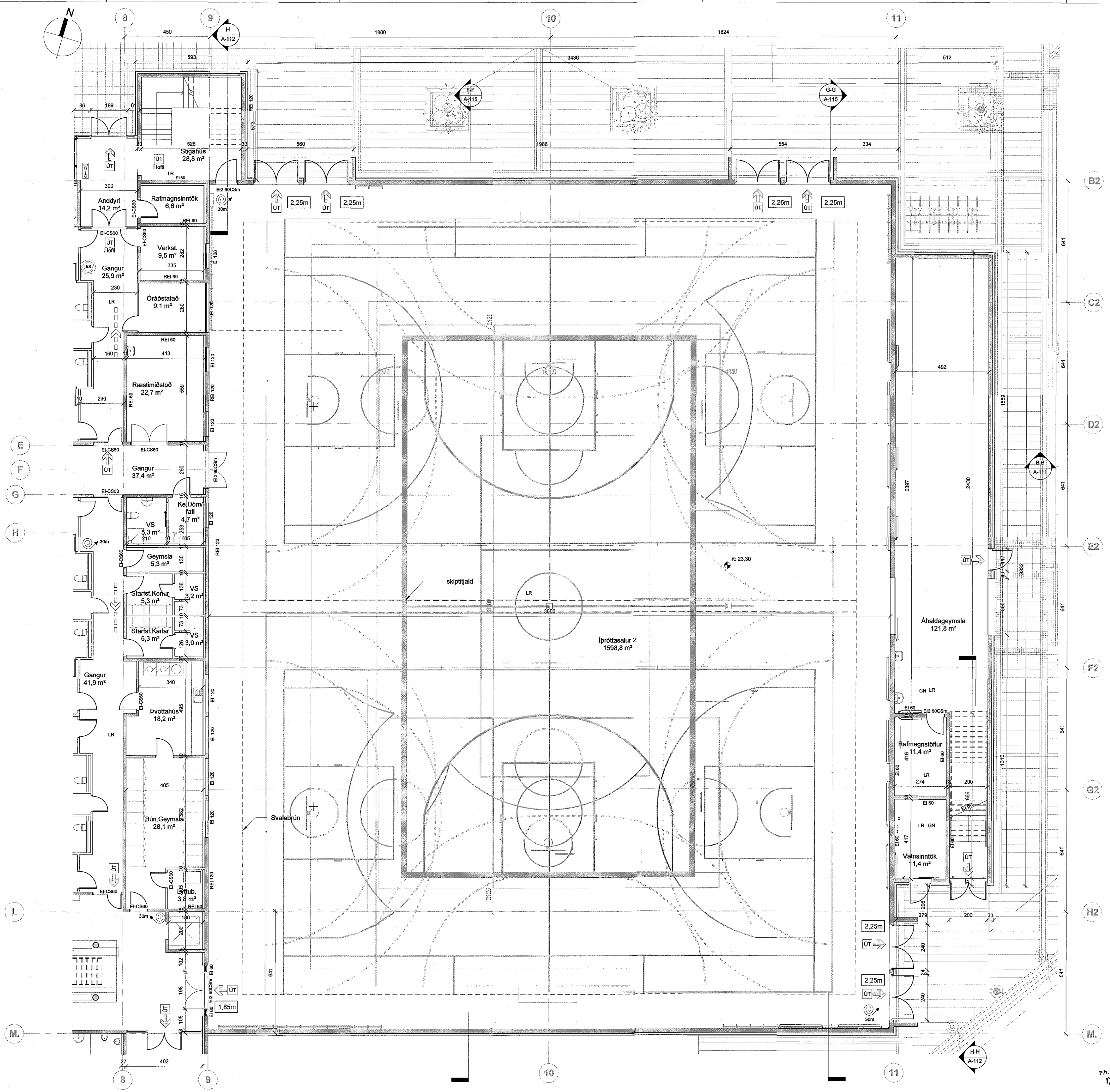
Hæð 1 - NA 1 : 100
