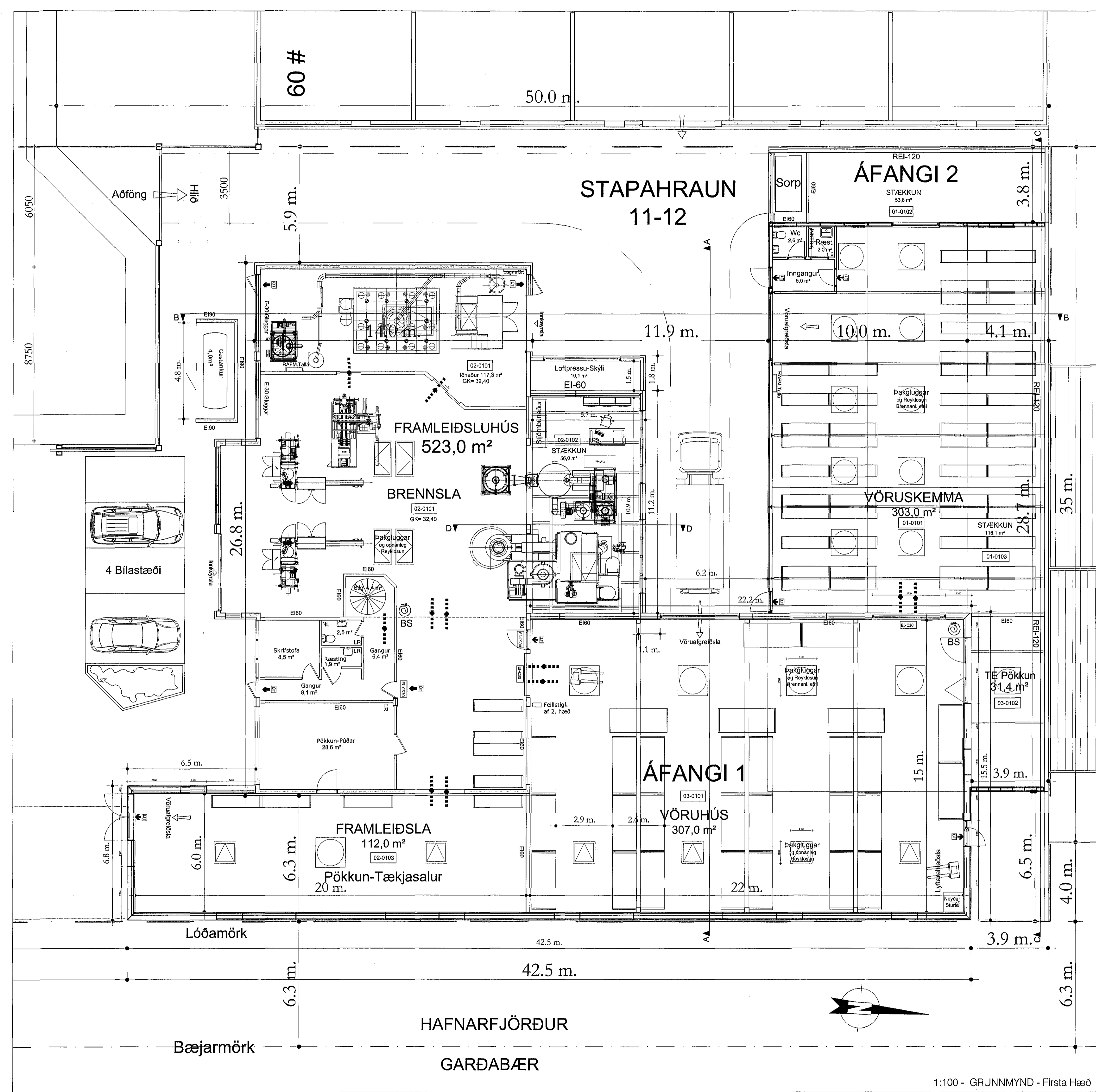
1:100 - GRUNNMÝND - Fírsta Hæð
