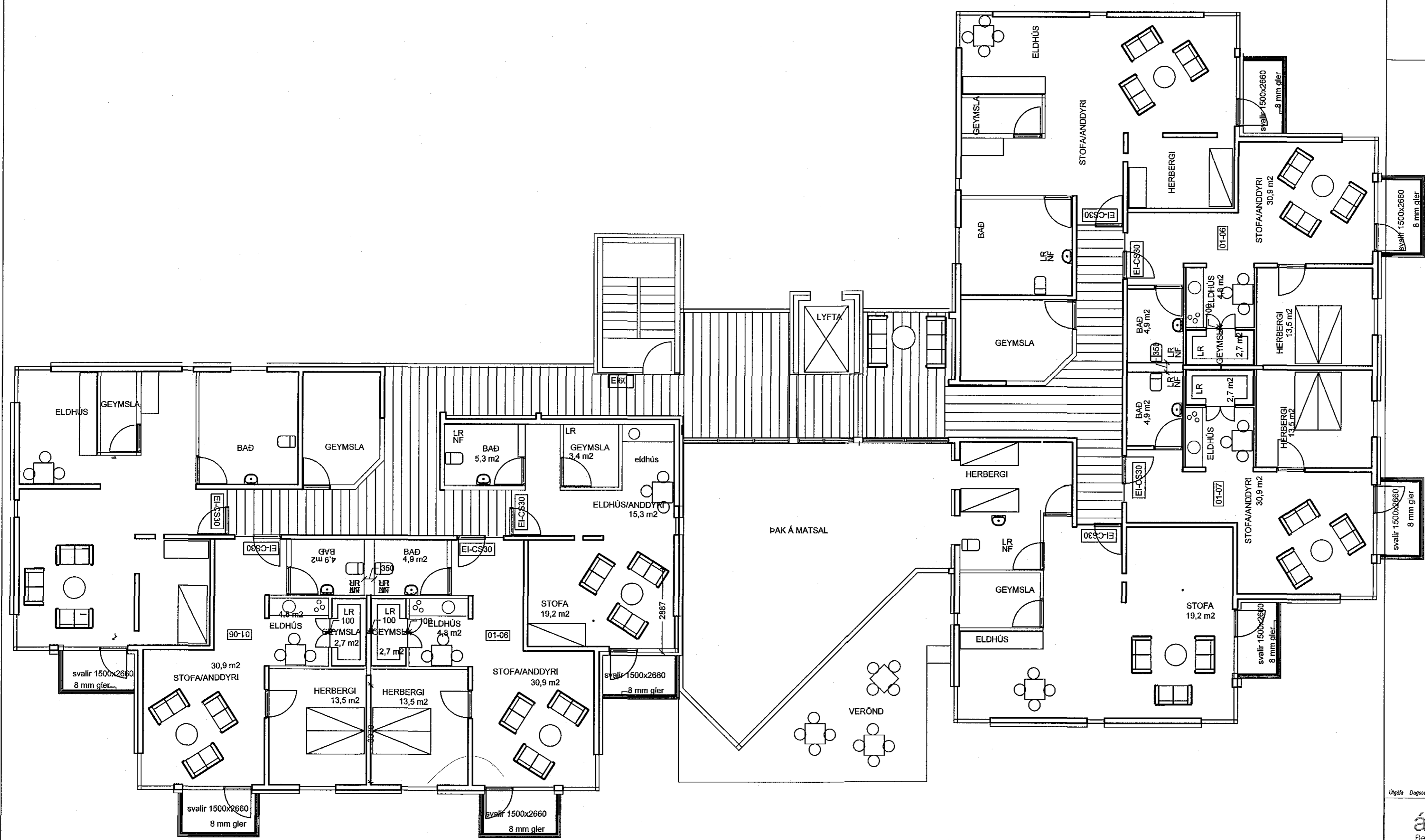
GRUNNMYND 2,3, og4 hæð og5.
